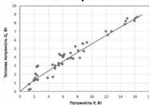
Рисунок 3 – Залежність теплової потужності від потужності установки
