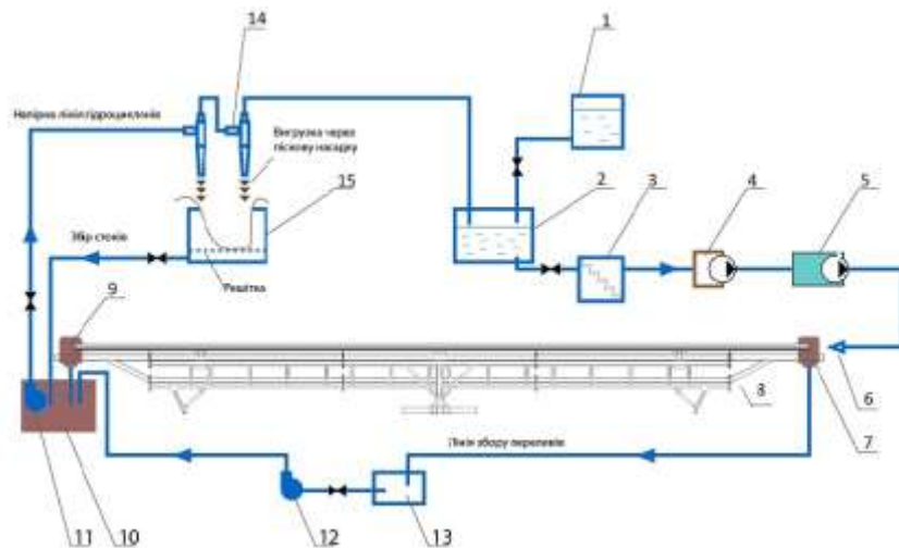
Рисунок 1 – Блок-схема дослідницької установки очищення насосно-компресорних труб, забруднених сольовими відкладеннями з умістом природних радіонуклідів комплексним методом:
