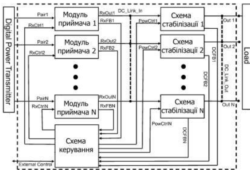
Рисунок 3 – Структурна схема системи цифрової передачі електроенергії багатоканальна
