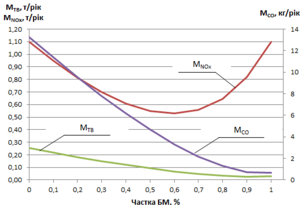
Рисунок 2 – Валові викиди оксидів азоту, оксиду вуглецю та твердих частинок у залежності від частки біомаси в суміші
