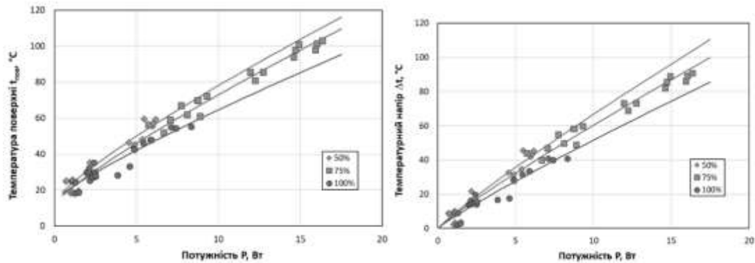
Рисунок 2 – Залежність температури поверхні трубки (а) та температурного напору (б) від потужності при різному вмісті графіту в матеріалі
