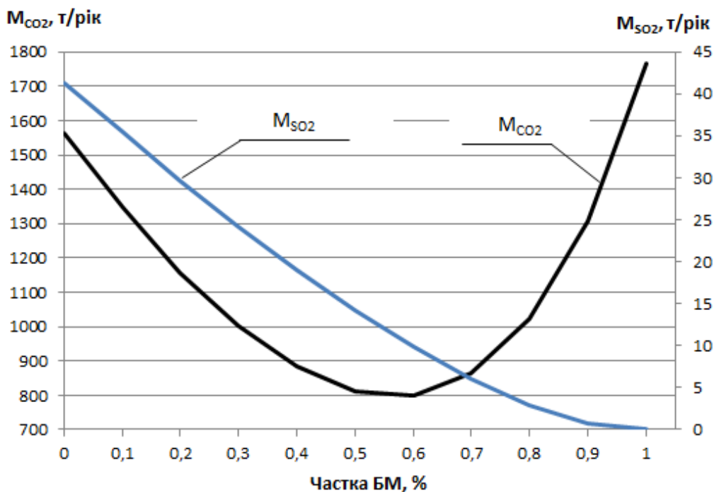
Рисунок 3 – Валові викиди діоксидів вуглецю та сірки в залежності від частки біомаси в суміші
