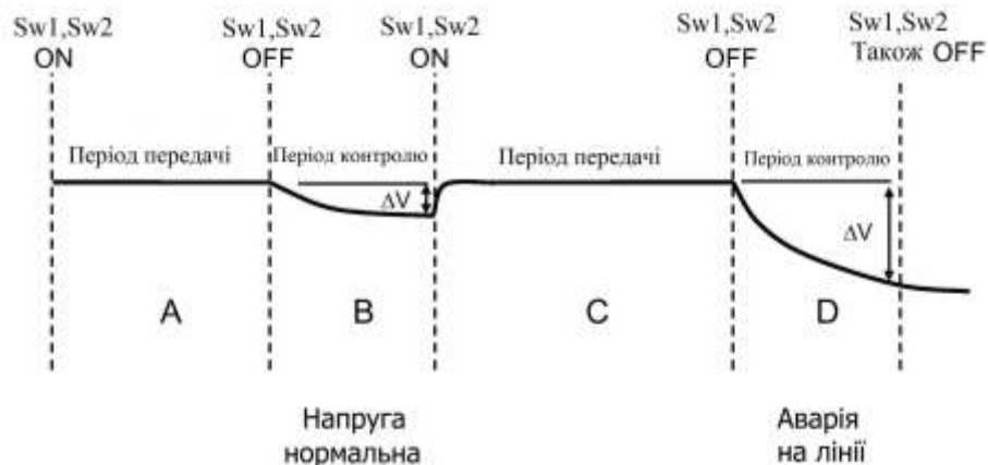
Рисунок 2 – Основні режими цифрової передачі електроенергії
