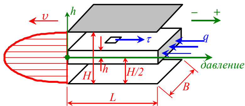
Рисунок 1 – Розрахункова схема плинущу матеріалу через канал
