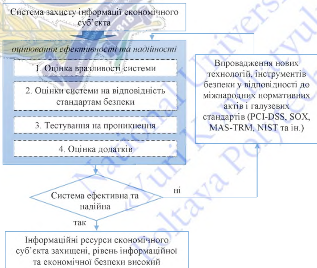
Рис. 3.4. Алгоритм побудови ефективної системи захисту інформації
