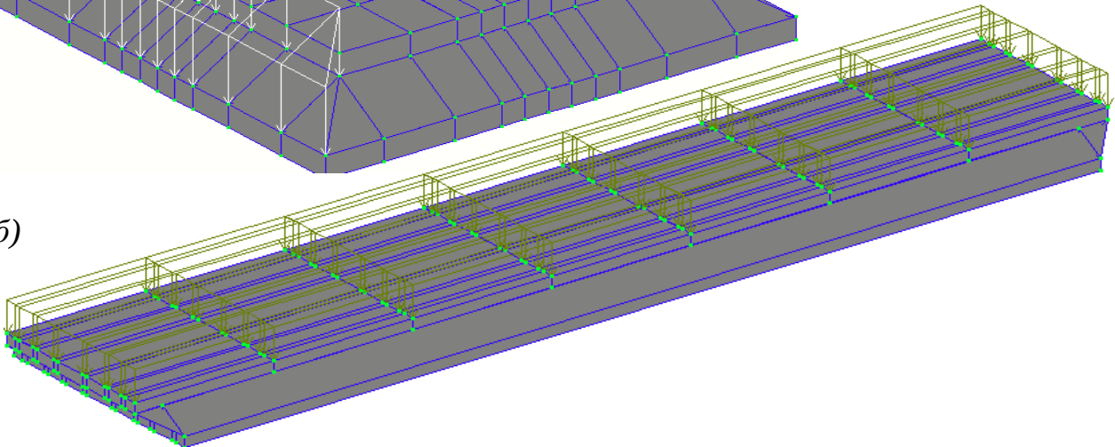
Рис. 12. Загальний вигляд кінцево-елементних моделей плит із прикладеним зовнішнім навантаженням:
