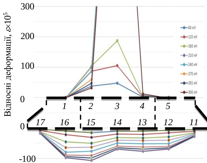
Рис. 5. Розподіл відносних деформацій на верхній (1 – 5) та нижній (11 – 17) поверхні зразка серії ПНК залежно від величини навантаження
