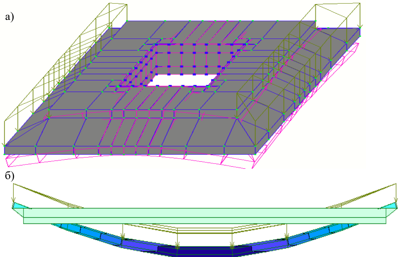
Рис. 13. Загальний деформований стан дослідних плит: а – надколонна плита; б – міжколонна плита
