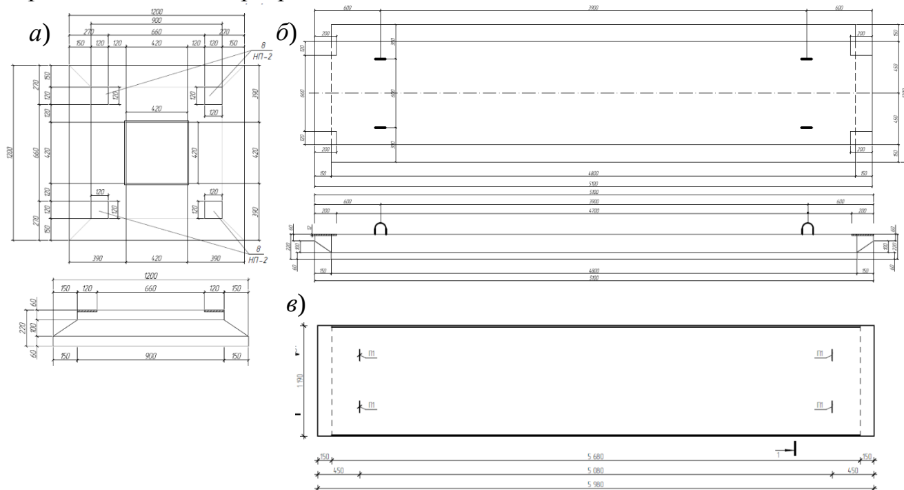
Рис. 3. Креслення досліджуваних плит: а – надколонна; б – міжколонна; в – пролітна
