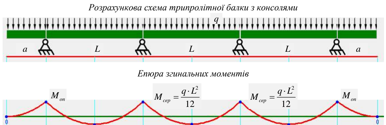
Рис. 5.3 – До визначення довжин консолей трипролітної балки
