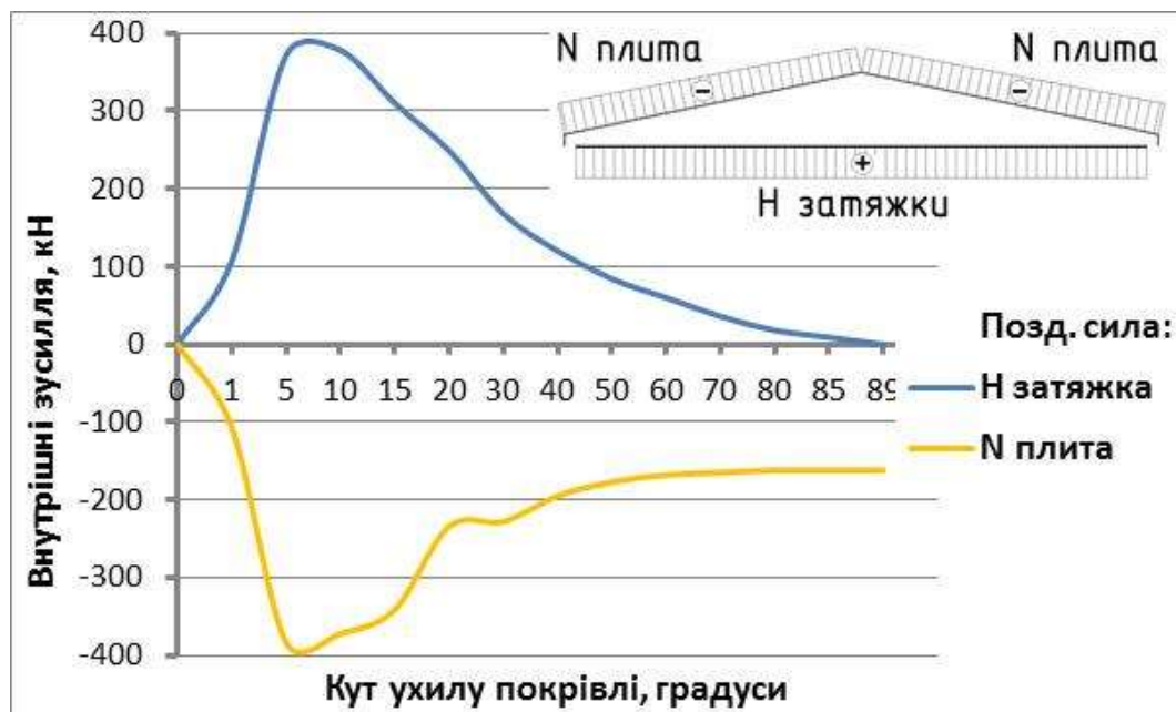
Рис. 6.10 – Графік зміни поздовжньої сили у перерізах сталеву затяжки та залізобетонної плити в залежності від ухилу покрівлі
