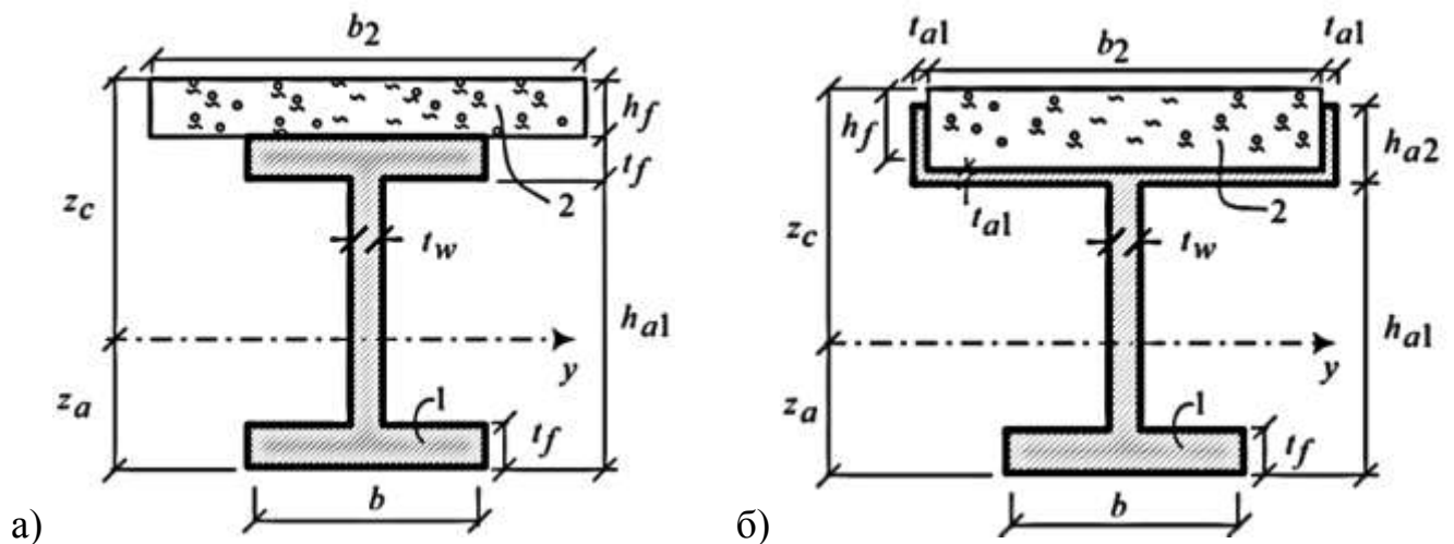
Рис. 1.16 – Переріз СЗБ балки [108]: а) типовий із прокатного профілю (1) і з/б плити (2); б) раціоналізований із тонкостінного «корита» з бетонною плитою (2)
