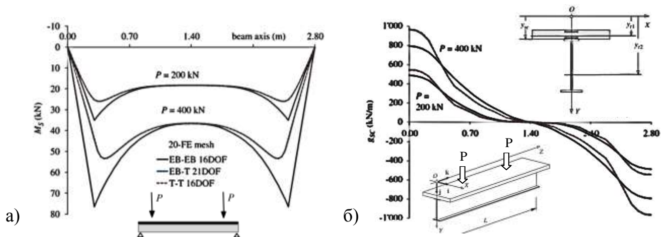
Рис. 1.17 – Графіки розподілу по довжині конструкції [234]: а) згинаючого моменту у сталевій частині; б) зсувного зусилля у контактному шві
