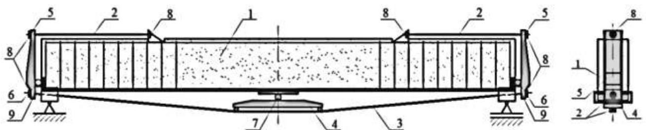
Рис. 1.3 – Загальний вигляд залізобетонної балки, підсиленої важільно-стрижневою системою [219]: 1 – залізобетонна балка; 2 – розтяжка; 3 – зтяжка; 4 – траверса; 5 – двоплечові важелі; 6,7 – котки; 8 –кріплення зі сферичними шайбами; 9 – упор
