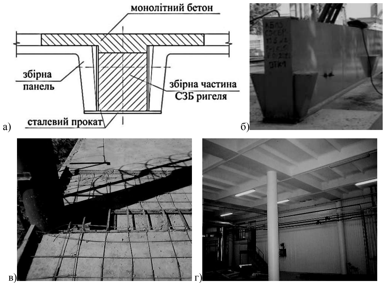
Рис. 1.13 – Збірно-монолітні сталезалізобетонні ригелі [13-14]:
