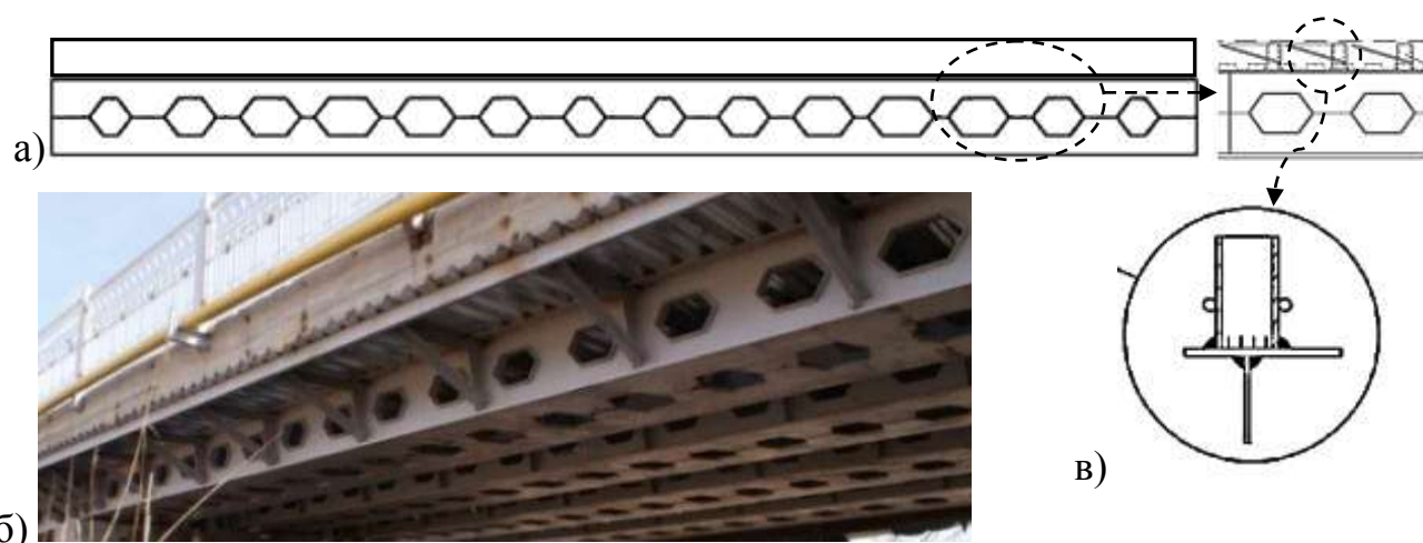
Рис. 1.18 – Схема (а) і загальний вигляд (б) перфорованих балок СЗБ оболонкових прогонових будов мостів; в) вузол поєднання металевих блоків і з/б плити [242]
