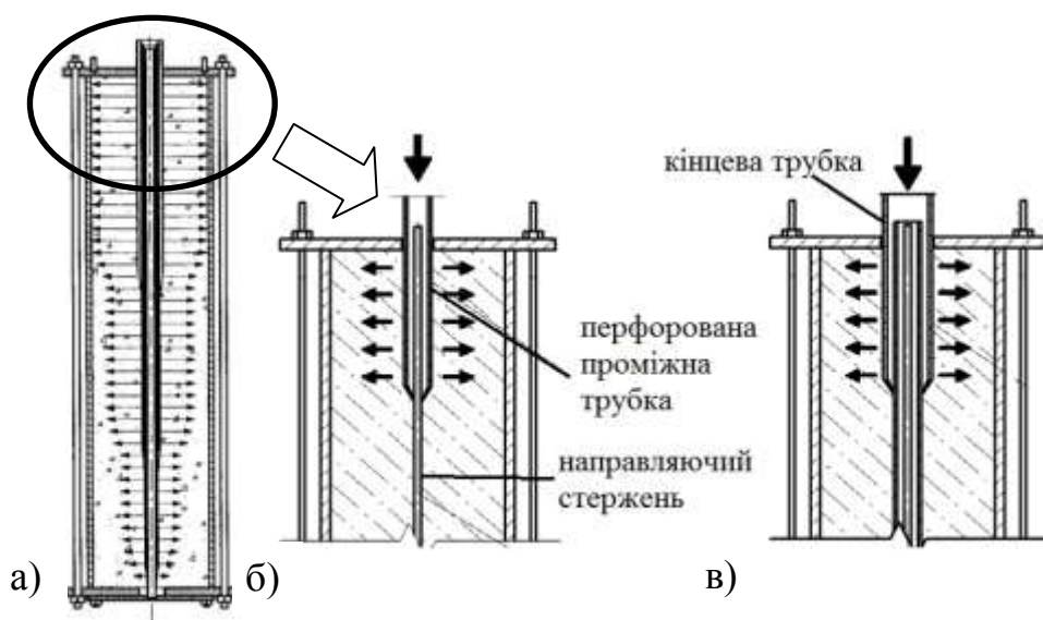
Рис. 1.28 – Зразки з попереднім обтиском бетонного ядра під час виготовлення [119]
