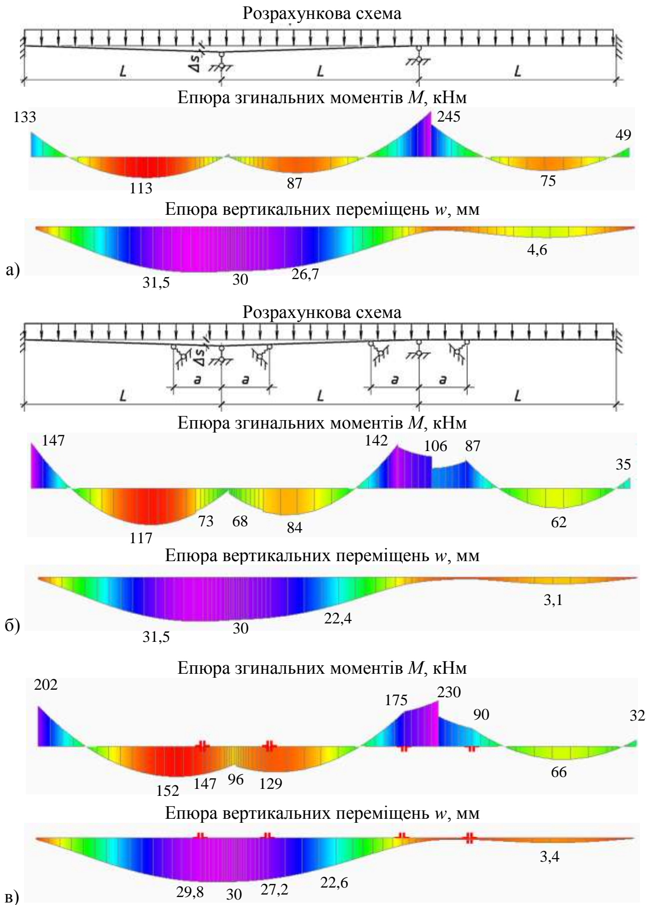
Рис. 7.17 – Епюри внутрішніх зусиль та переміщень балок сталезалізобетонного перекриття для розрахункових випадків: а) Г.2.1; б) Г.2.21; в) Г.2.2.2
