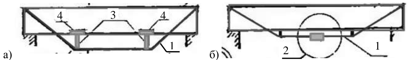
Рис. 1.6 – Типові конструктивні рішення [134] зовнішнього підсилення залізобетонних конструкцій сталевими тяжами (шпренгелями) (поз. 1) із натягом останніх шляхом: а) підклинюванням сталевими пластинами (поз. 3-4); б) стяжною муфтою (поз. 2)
