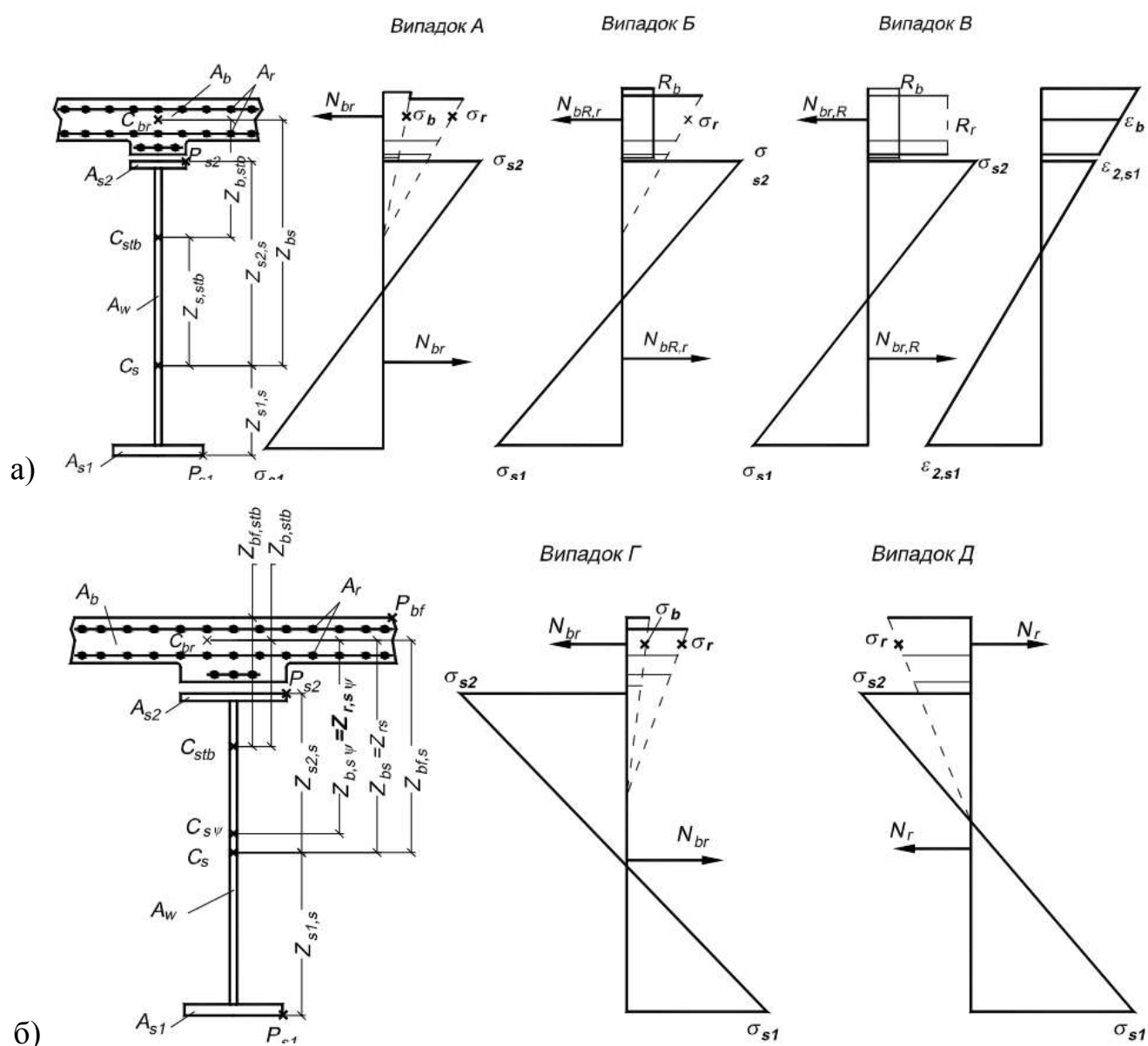
Рис. 1.40 – Зусилля, напруження і деформації в СЗБ поперечному перерізі, що сприймає додатній (а) чи від'ємний (б) згинальні моменти [77]
