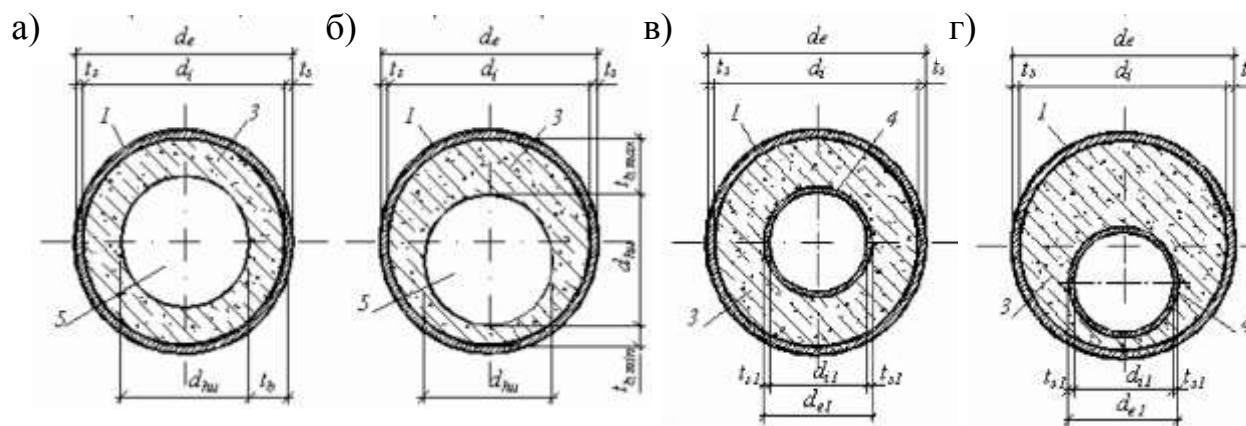
Рис. 1.27 – Перерізи трубобетонних елементів із центрифугованим бетонним осердям [94]: 1 – сталева зовнішня труба-оболонка; 3 – центрифугований бетон; 4 – внутрішня труба; 5 – внутрішня порожнина
