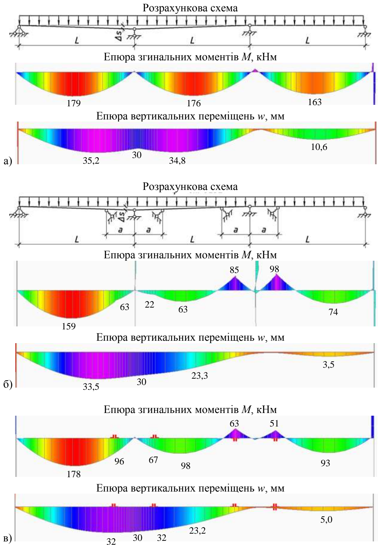
Рис. 7.16 – Епюри внутрішніх зусиль та переміщень балок сталезалізобетонного перекриття для розрахункових випадків: а) В.2.1; б) В.2.21; в) В.2.2.2
