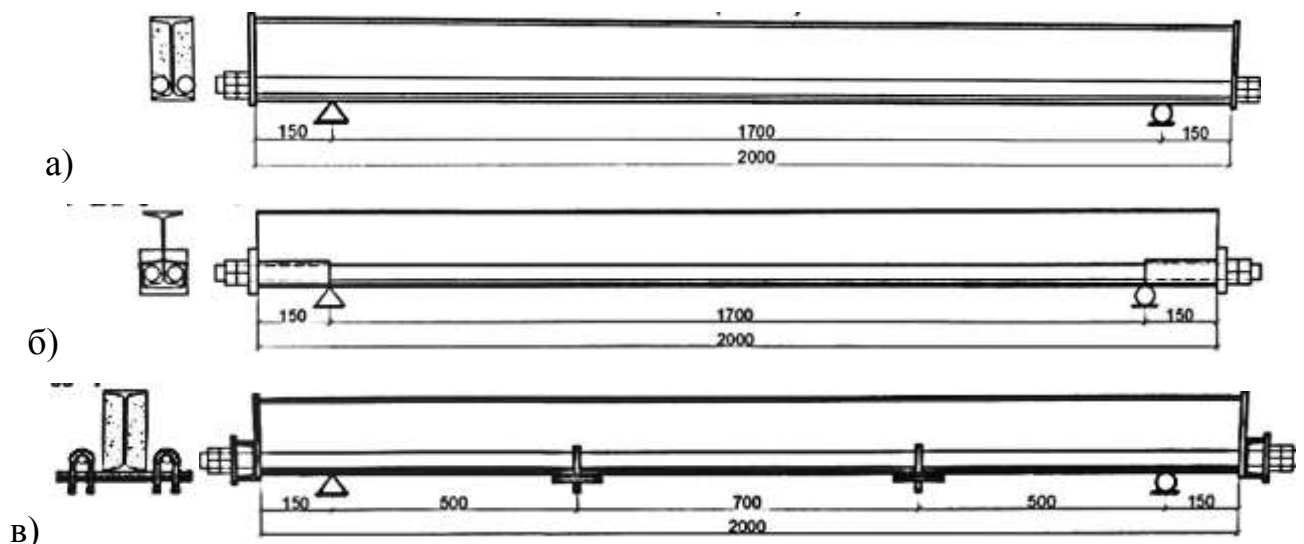
Рис. 1.10 – Схеми додаткового попередньо напруженого внутрішнього (а-б) та зовнішнього (в) армування сталобетонних балок [124]
