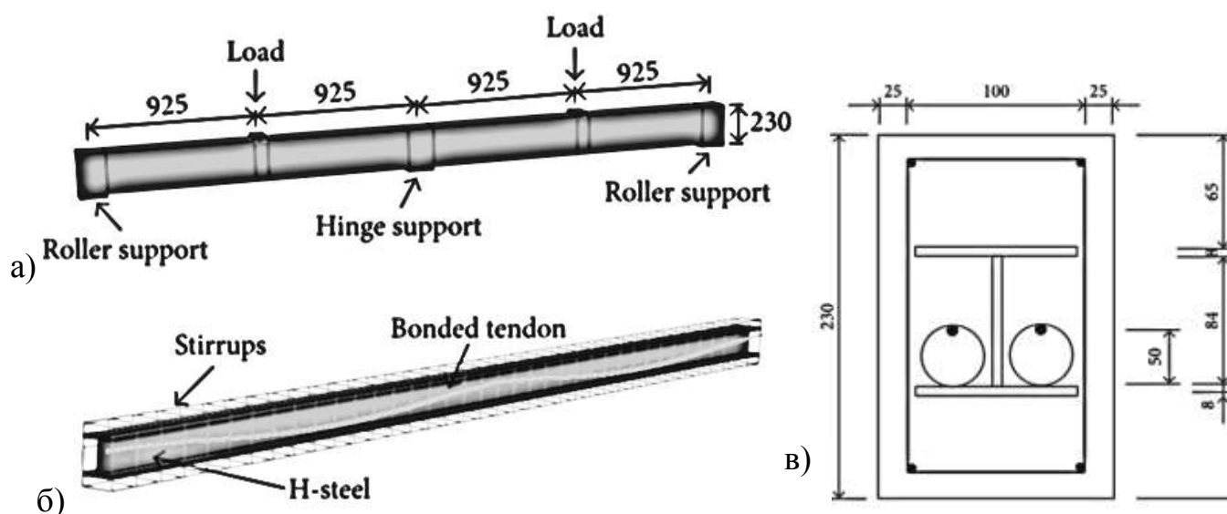
Рис. 1.11 – Попередньо напружені сталезалізобетонні балки [353]:
