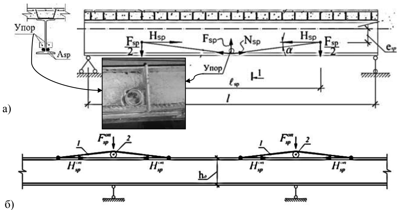
Рис. 1.7 – Влаштування напружуваних арматурних стержнів сталезалізобетонних балок [101]: а) загально в пролітній частині розрізної балки; б) локально на проміжних опорах нерозрізної балки; 1 – затяжка; 2 – упорний циліндр
