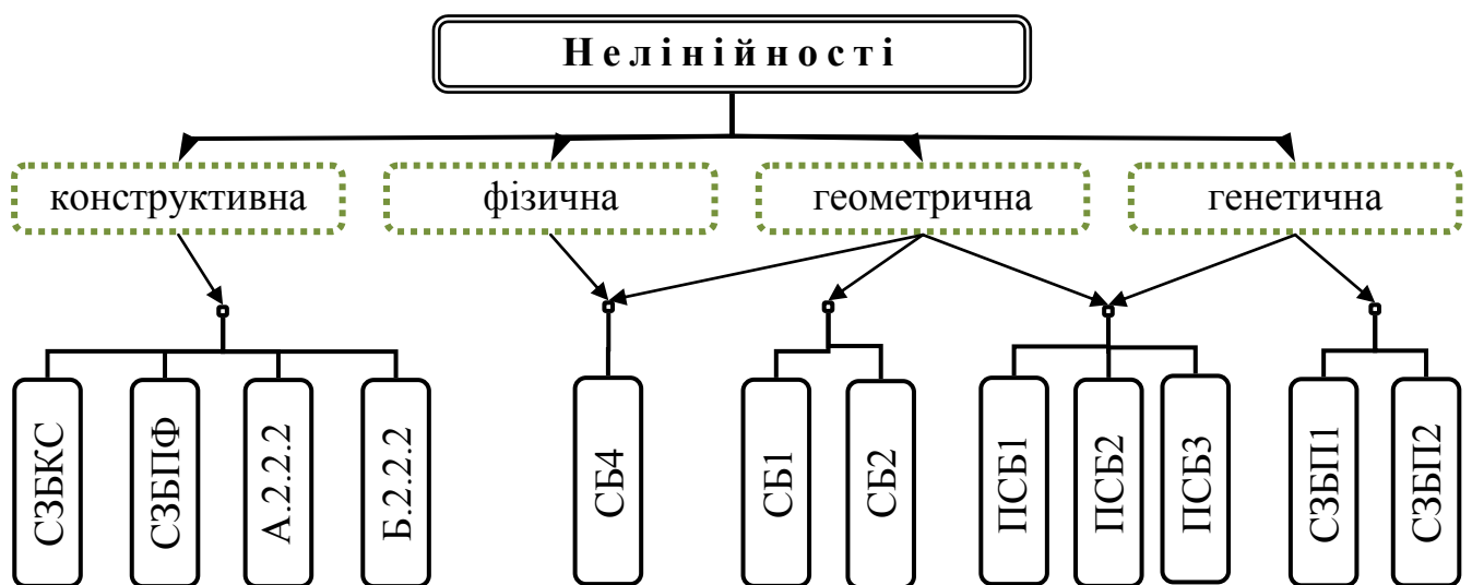
Рис. 7.24 – Класифікація самонапружених СЗБК від типу дослідженої нелінійності
