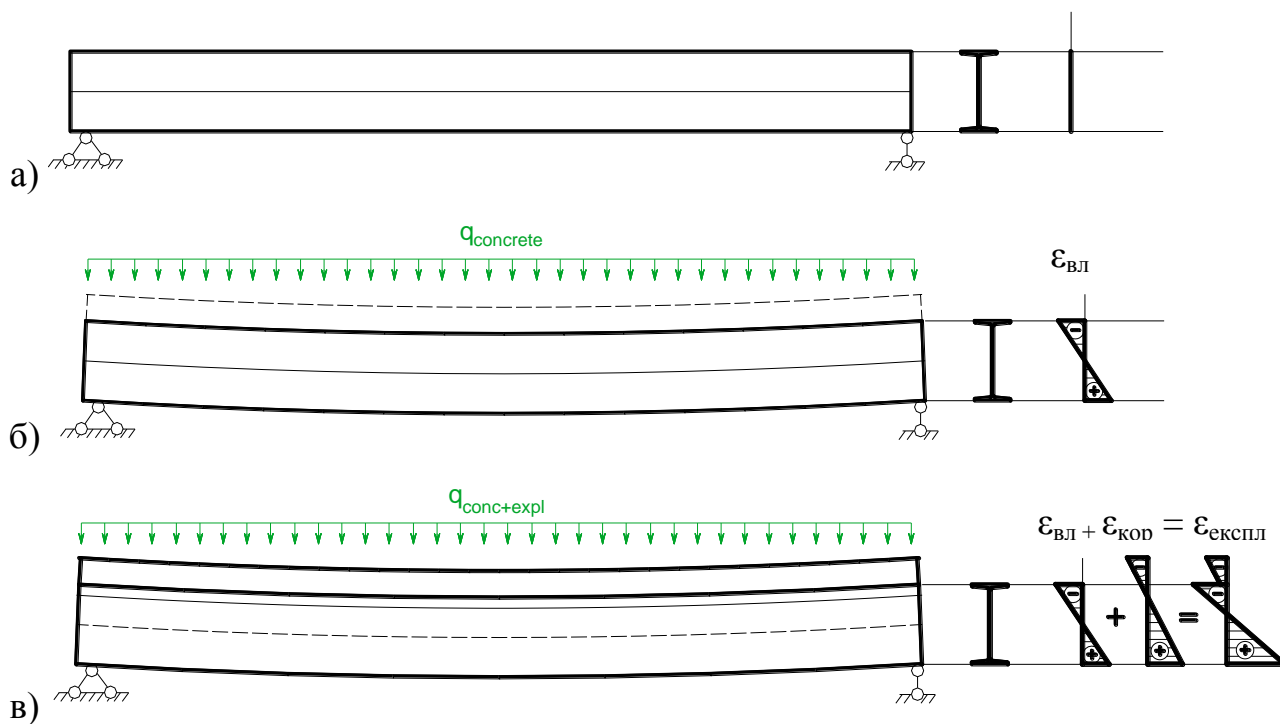
Рис. 4.2 – Стадії роботи комбінованого сталезалізобетонного перекриття, виготовленого за двостадійною технологією: а) монтаж сталевих балок; б) влаштування монолітної плити перекриття; в) експлуатаційна стадія
