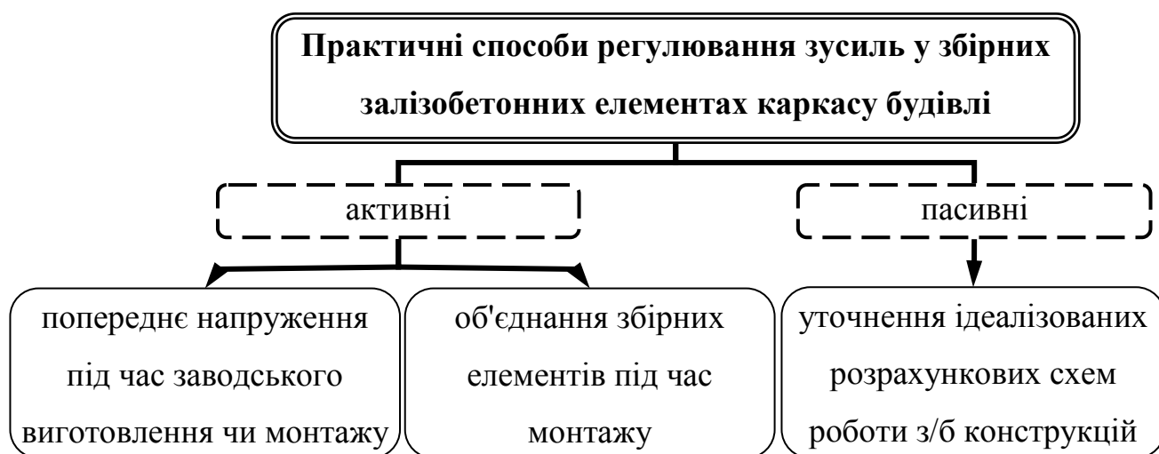
Рис. 1.32 – Способи регулювання зусиль у збірних залізобетонних конструкціях
