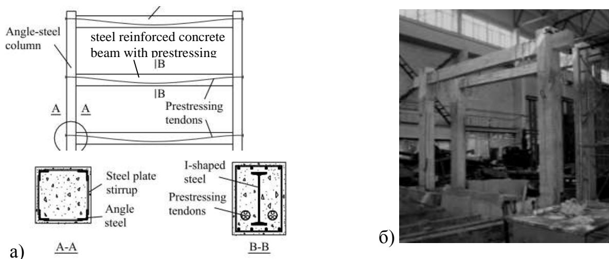
Рис. 1.12 – Досліджені рами [354]: а) схема елементів; б) загальний вигляд
