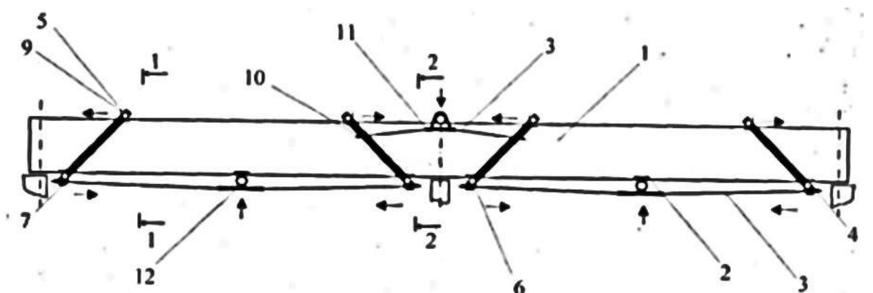
Рис. 1.5 – Система зовнішнього підсилення залізобетонних нерозрізних балок [214]: 1 – з/б балка; 2 – закладні пластини; 3 – з'язки; 4 – анкери; 5, 6 – верхній і нижній стержні; 7 – поздовжнє плече; 8 – отвір для закріплення з'язки; 9, 10 – упори; 11 – траверса над опорою; 12 – траверса в прольоті балки
