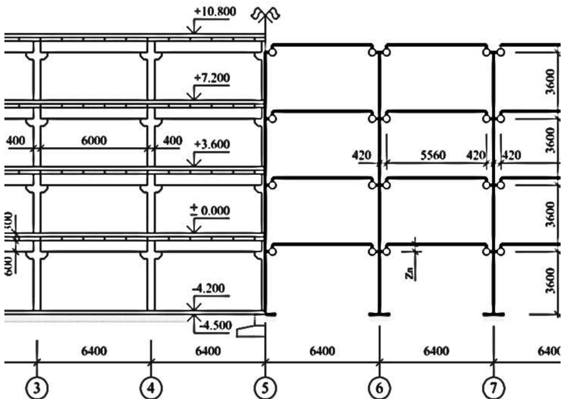
Рис. 1.37 – Схематичне креслення та розрахункова схема із П-подібною формою ригеля фрагменту поперечної рами будівля [110]
