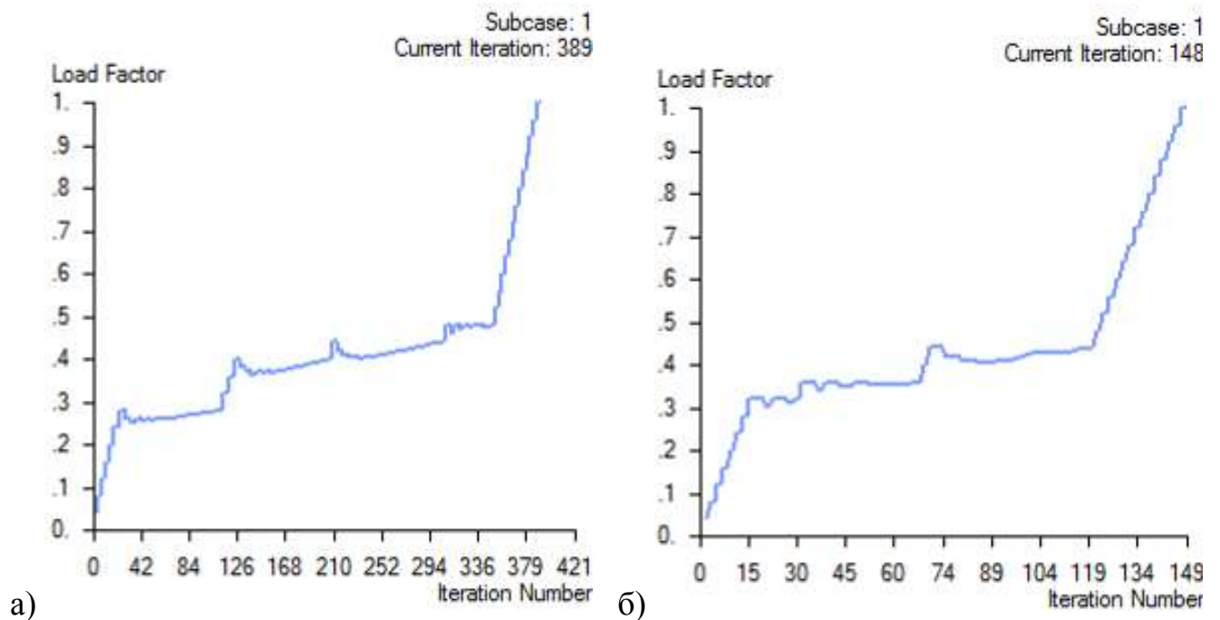
Рис. 7.15 – Графічна інтерпретація ходу розрахунку підсилюваних сталевих балок при шарнірному (а) та жорсткому (б) вузлі їх примикання до колон
