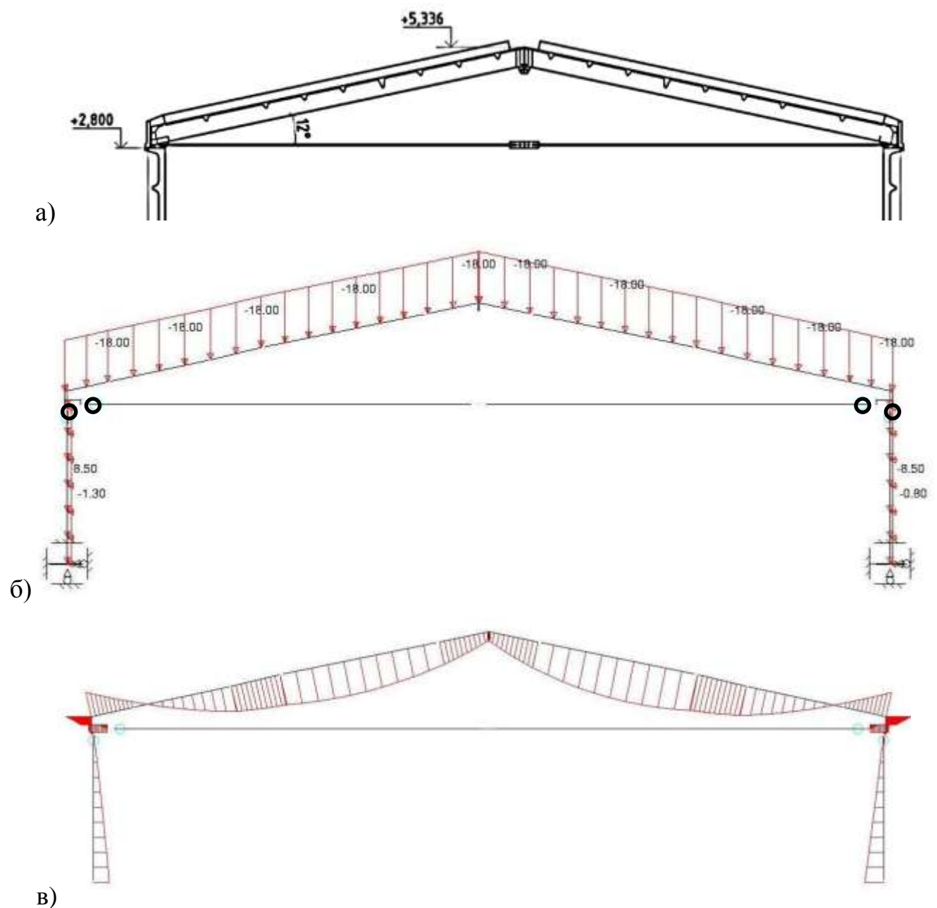
Рис. 6.20 – Експлуатаційне положення плити: а) схематичне креслення; б) розрахункова схема; в) епюра згинальних моментів, кНм
