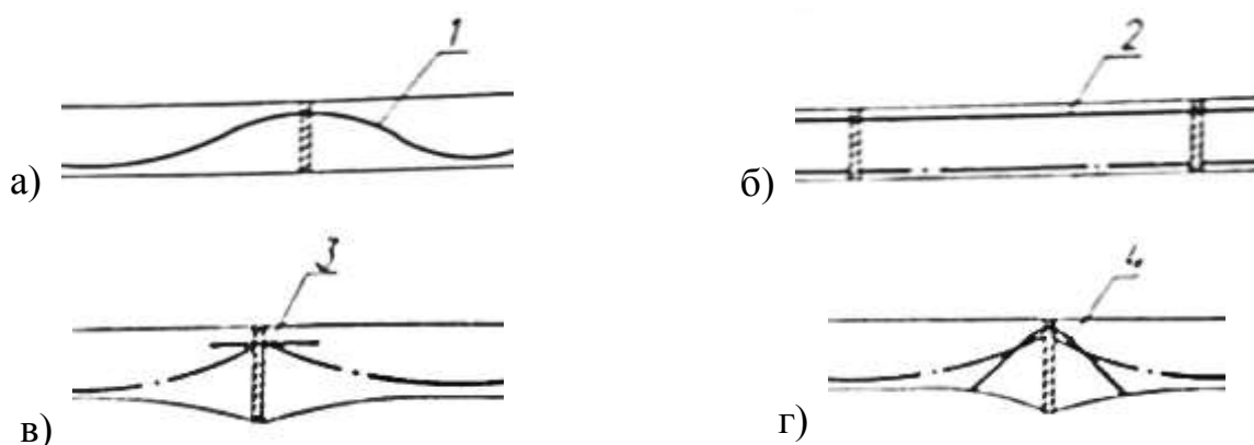
Рис. 1.35 – Фрагменти надпорних вузлів попередньо напружених стиків збірно-монолітних залізобетонних конструкцій [58]
