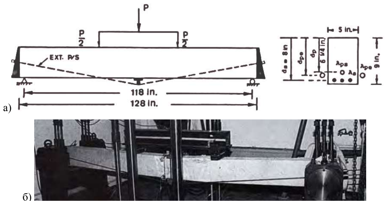
Рис. 1.9 – Розміри (а) та загальний вигляд (б) залізобетонних балок, підсилених зовнішнім стрижневим армуванням [312]
