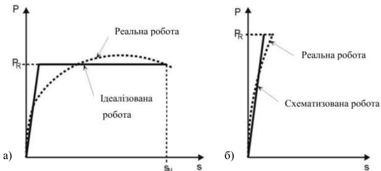
Рис. 1.42 – Характер роботи гнучких (а) і жорстких (б) анкерів [88]
