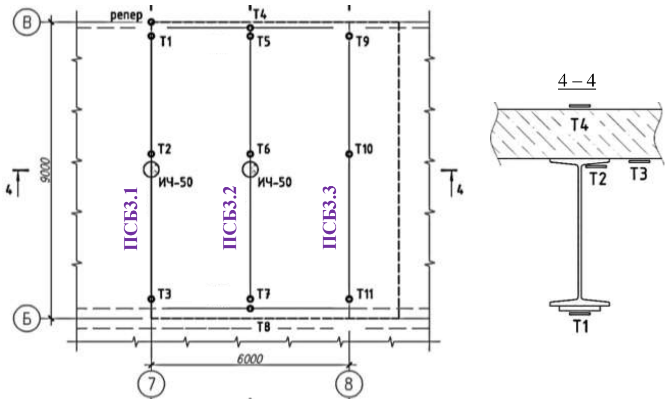
Рис. 4.32 – Схема розміщення контрольних точок нівелювання, індикаторів годинникового типу ІЧ-50 та електротензорезисторів
