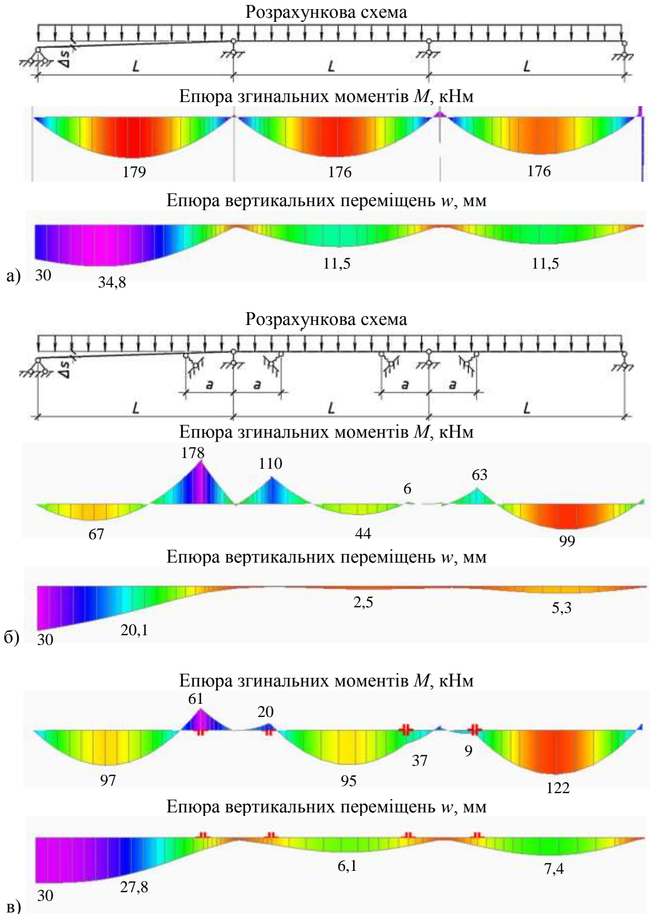
Рис. 7.18 – Епюри внутрішніх зусиль та переміщень балок сталезалізобетонного перекриття для розрахункових випадків: а) Д.2.1; б) Д.2.21; в) Д.2.2.2
