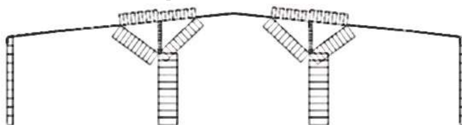
Рис. 2.12 – Розрахункова схема та епюри внутрішніх зусиль у поперечній трипролітній рамі будівлі з підкосами
