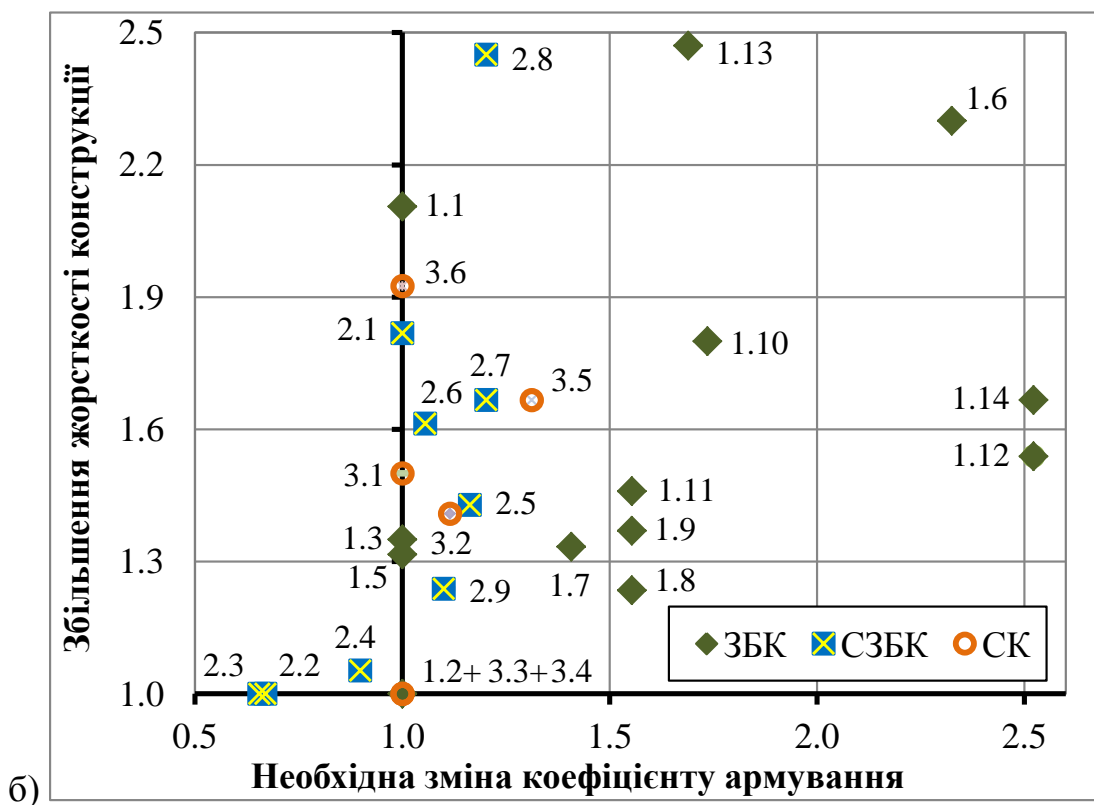
Рис. 2.2 – Збільшення несучої здатності (а) та жорсткості (б) будівельних конструкцій в залежності від зміни коефіцієнту армування, необхідного для раціонального регулювання зусиль в них
