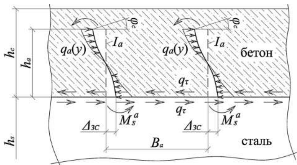
Рис. 3.7 – Фрагмент сталевих і бетонних шарів при їх відносному зсуві на величину \Delta_{зс} та анкерних засобів між ними ( I_c, I_s, I_a – моменти інерції відповідно бетонного і сталевих шарів та анкерних засобів у площині їх згину)
