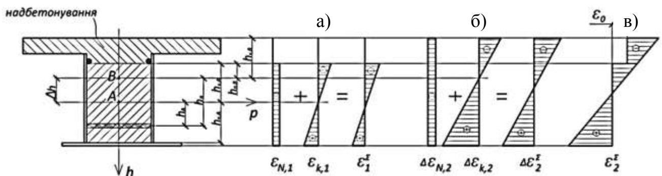
Рис. 1.14 – Епюри відносних деформацій у сталезалізобетонному ригелі [174]:
