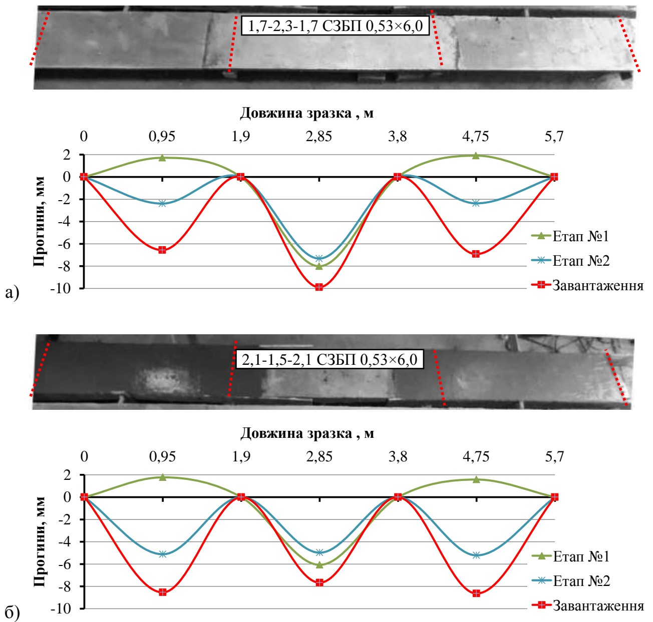
Рис. 5.33 – Зміна прогинів в кінці двох етапів бетонування та при максимальному завантаженні зразків: а) 1,7-2,3-1,7 СЗБП 0,53×6,0; б) 2,1-1,5-2,1 СЗБП 0,53×6,0
