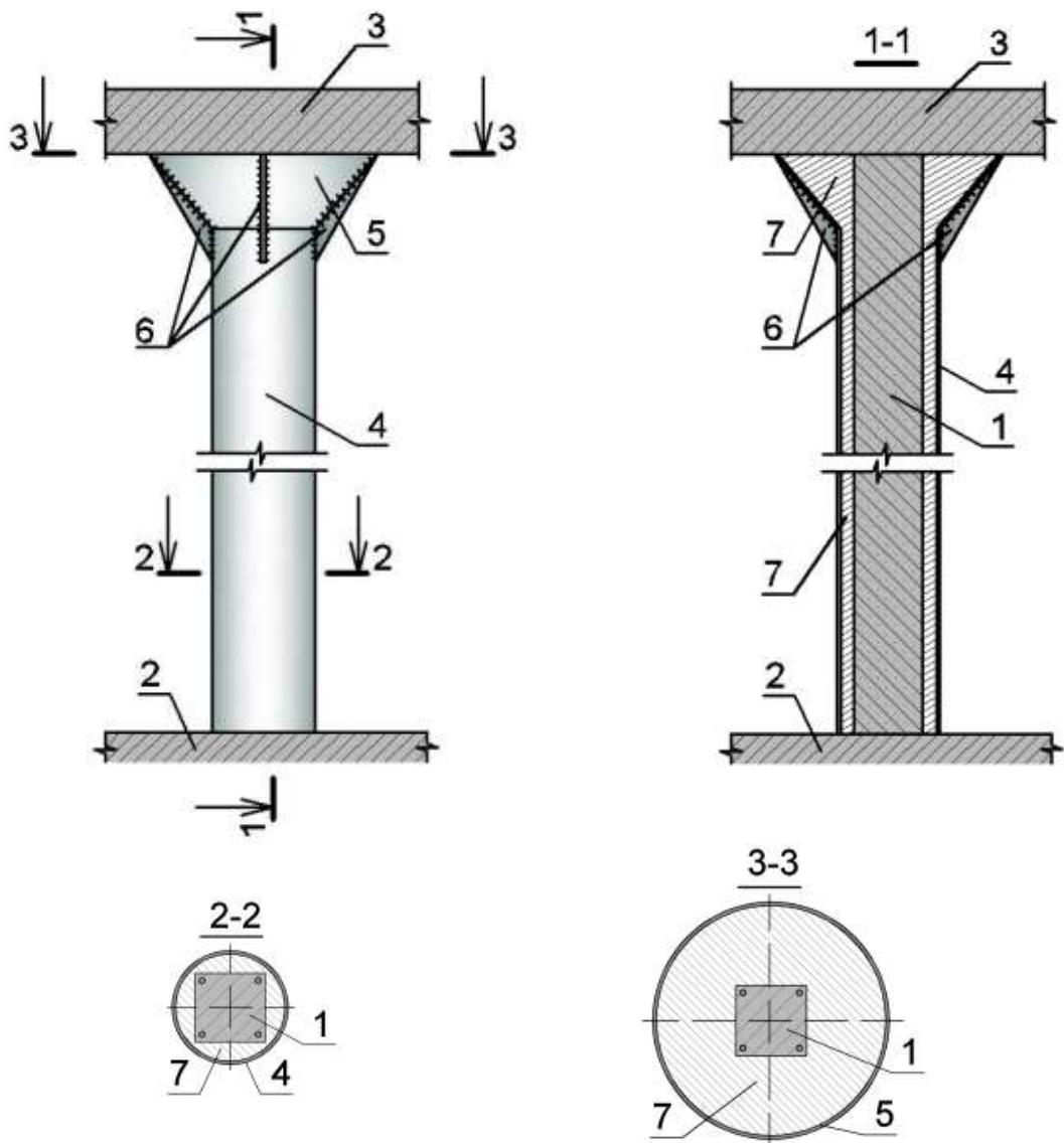
Рис. 7.22 – Спосіб підсилення пошкодженої залізобетонної колони сталеву обоймою із включенням її в сумісну роботу
