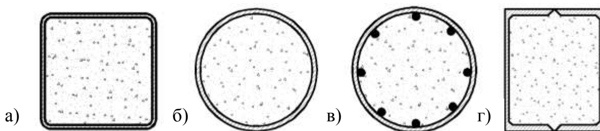
Рис. 1.26 – Перерізи трубобетонних елементів [266]: а-б) з квадратних та круглих труб; в) з додатковою стержневою арматурою; г) зі швелерів, з'єднаних «в короб»
