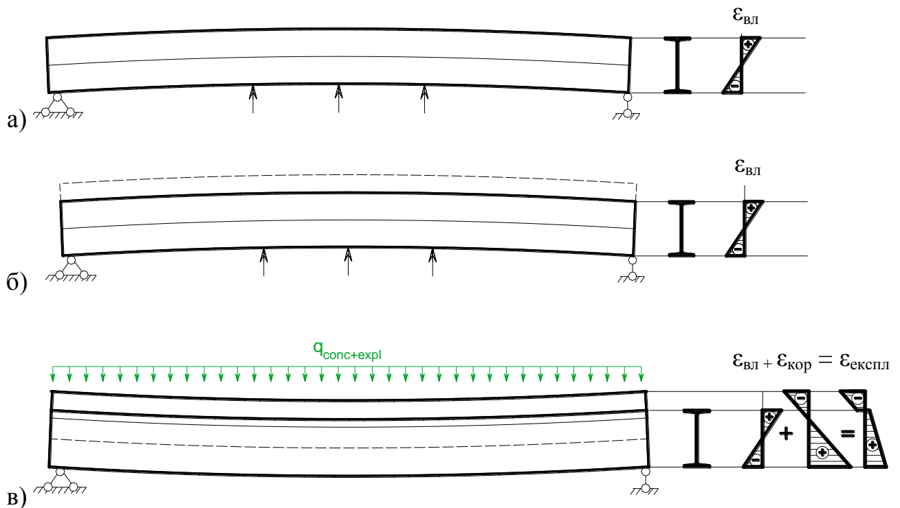
Рис. 4.3 – Стадії роботи комбінованого попередньо напруженого сталезалізобетонного перекриття: а) монтаж сталевих балок та створення їх попереднього вигину; б) влаштування монолітного залізобетонного перекриття при наявності тимчасових стійок під сталевими балками; в) експлуатаційна стадія
