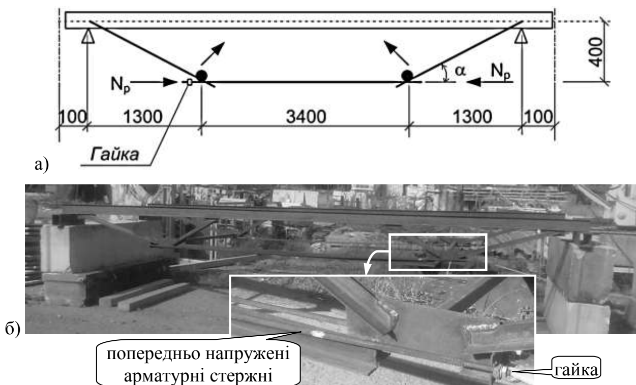
Рис. 1.23 – Створення зусиль натягу в зтяжці шпренгельної сталезалізобетонної конструкції [98]: а) схема; б) загальний вигляд натурної моделі
