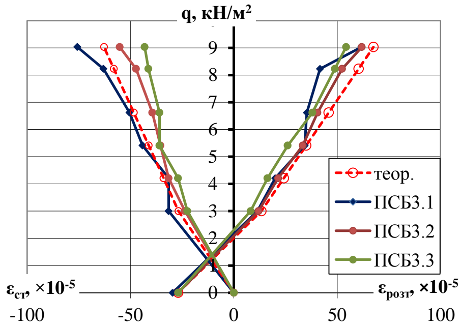
Рис. 4.33 – Приріст відносних деформацій найбільш стиснутого та розтягнутого волокон перерізу сталезалізобетонних балок серії ПСБЗ
