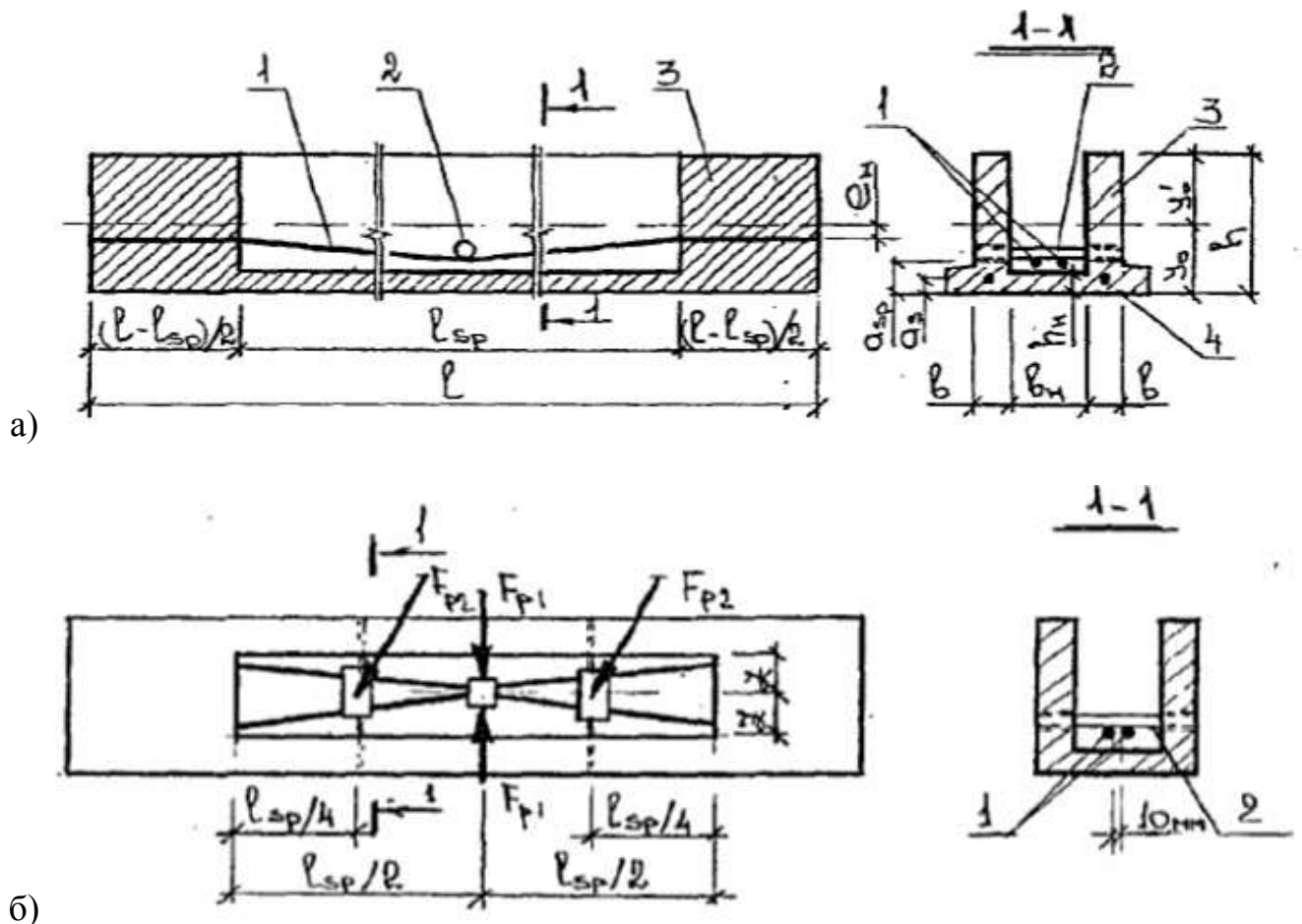
Рис. 1.8 – Локально попередньо напружена шпренгелем балка збірно-монолітного сталезалізобетонного перекриття [139]: а) будова; б) схема двохетапного натягу арматури; 1 – напружувана арматура; 2 – упорний стержень; 3 – залізобетонна частина балки; 4 – ненапружувана арматура
