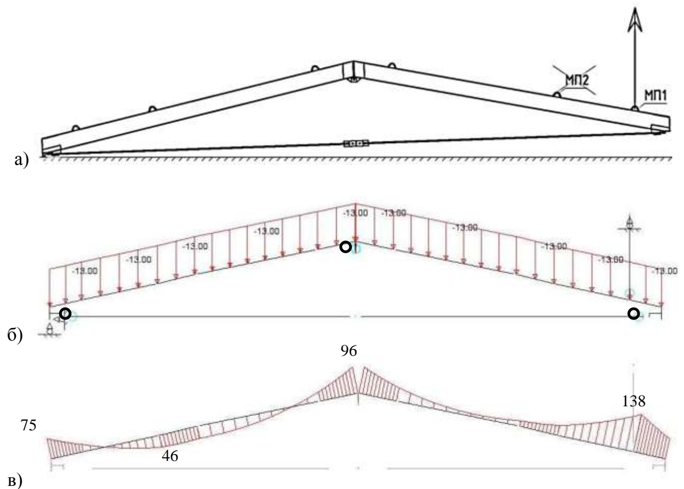
Рис. 6.17 – Підйом зібраної панелі із шарнірним гребеневим вузлом за дві крайні (ближчі до опор) монтажні петлі МП1: а) схема стропування; б) розрахункова схема; в) епюра згинальних моментів, кНм
