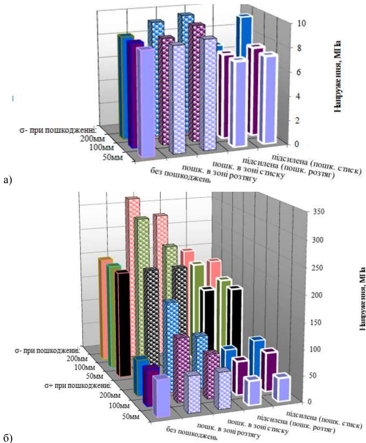
Рис. 2.23 – Зміна максимальних напружень у бетоні (а) та в стержнях арматури (б) залізобетонної колони в залежності від величини пошкодження
