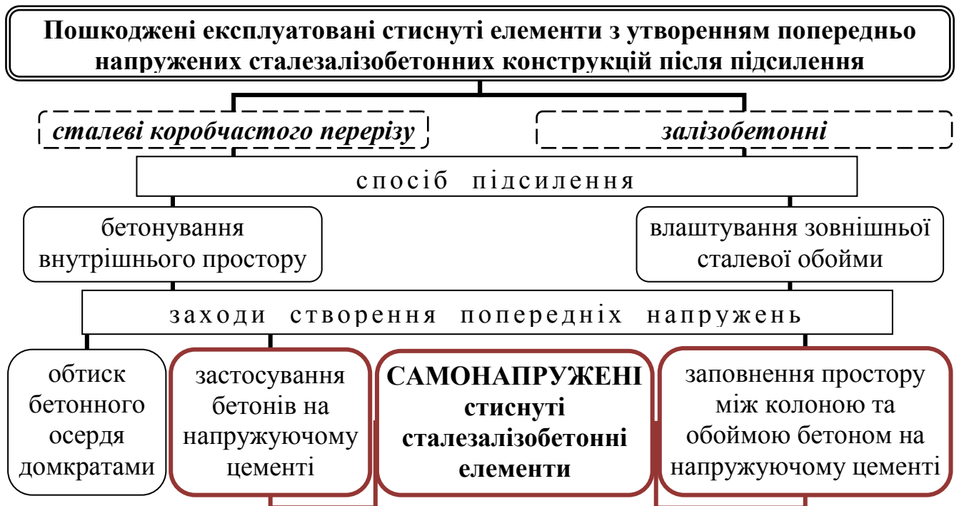
Рис. 7.23 – Заходи створення попередніх напружень в елементах підсилення експлуатованих стиснутих конструкцій
