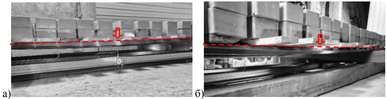
Рис. 5.22 – Прогини: а) 1/225 в крайньому прольоті зразка 1,9-1,9-1,9 K35-0,5 ( 118 \text{ кг/м}^2 ); б) 1/250 в середньому прольоті зразка 1,75-2,2-1,75 K35-0,5 ( 146 \text{ кг/м}^2 )
