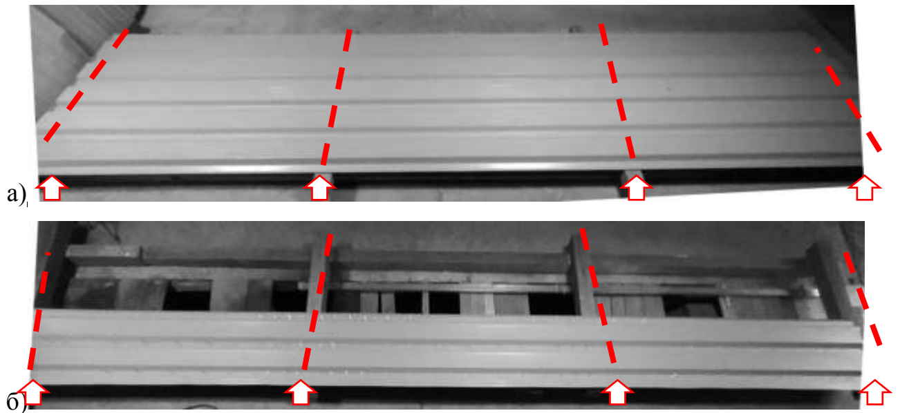
Рис. 5.15 – Загальний вигляд експериментально досліджених листів профільованого настилу марки К35-0,5 довжиною 6000 мм: а) шириною 1060 мм; б) шириною 530 мм
