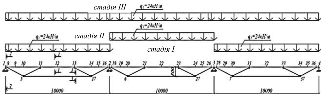
Рис. 1.24 – Схеми завантаження нерозрізної комбінованої конструкції [96; 97]
