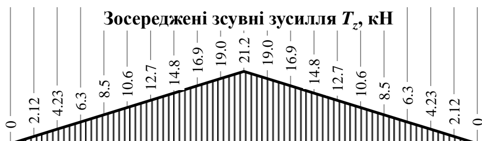
Рис. 3.18 – Епюри зсувних зусиль по довжині однопролітної сталезалізобетонної балки, завантаженої по центру прольоту зосередженою силою (серія СБ1)
