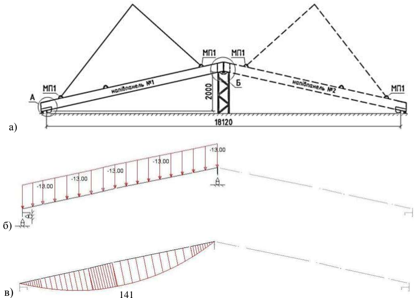
Рис. 6.15 – Встановлення двох напівпанелей на монтажні кондуктори для їх укрупнювальної збірки: а) схема встановлення; б) розрахункова схема; в) епюра згинальних моментів, кНм
