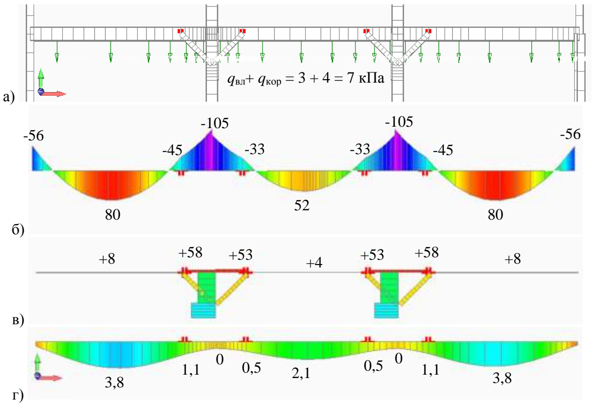
Рис. 7.14 – Розрахунковий випадок Б.2.2.2:
