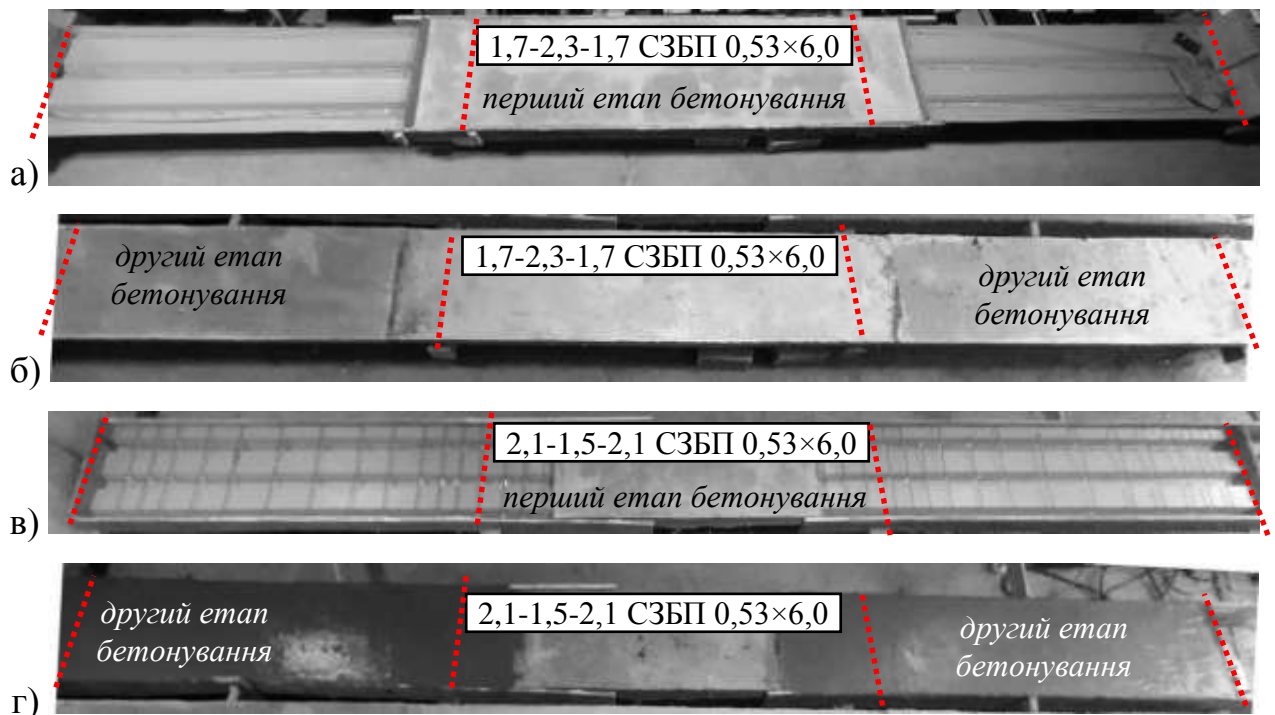
Рис. 5.29 – Загальний вигляд зразків сталобетонних плит на етапах бетонування
