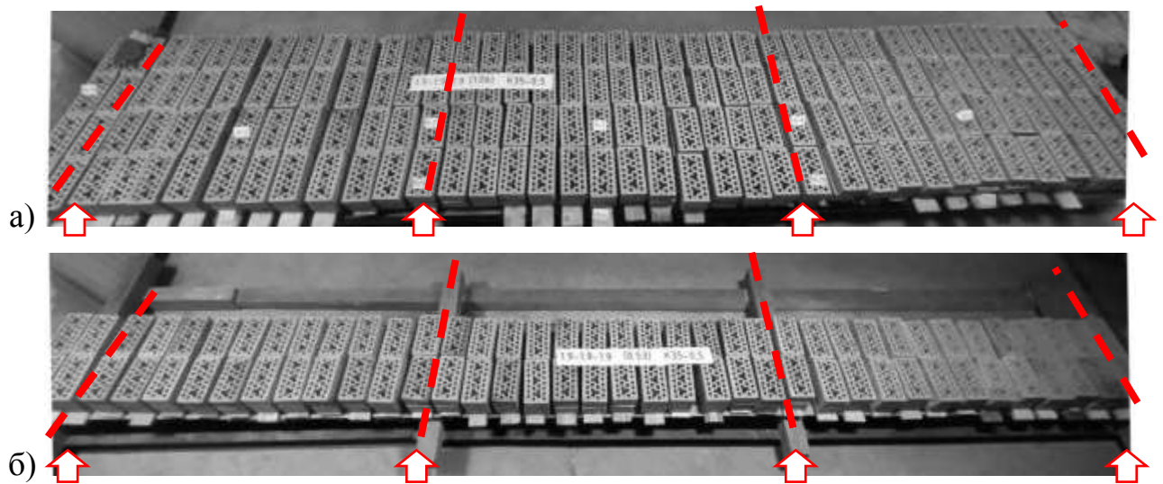
Рис. 5.18 – Загальний вигляд завантажених зразків профільованого настилу:
