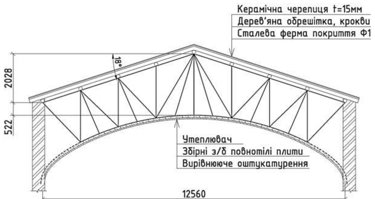
Рис. 6.23 – Схематичний поперечний розріз просторової системи покриття
