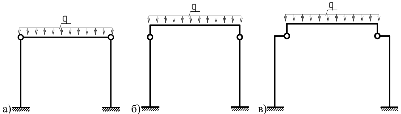
Рис. 1.36 – Розрахункові схеми однопролітних одноповерхових рам [55]: з шарнірним осьовим (а) та неосьовим (б-в) приєднання ригеля
