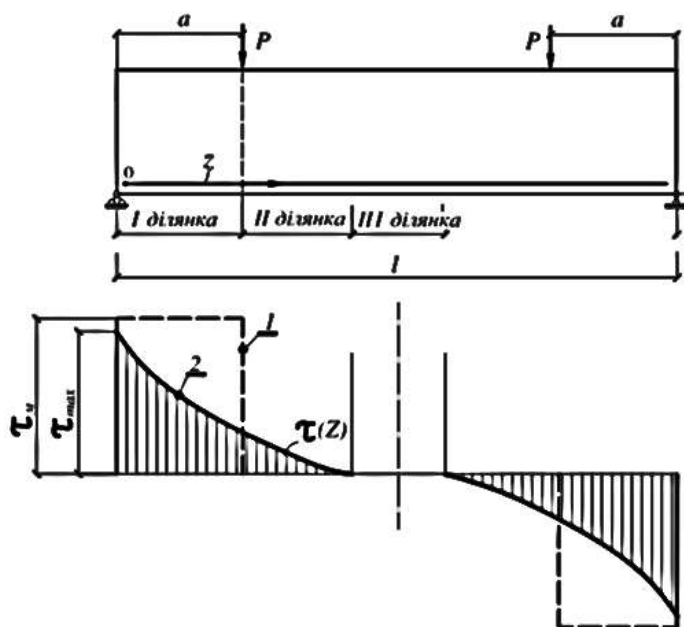
Рис. 1.47 – Уточнена еюра (поз.2) дотичних напружень (б) вздовж поверхні шва двокомпонентного ЗБЕ (а) при несумісності деформацій бетону і арматури [300]
