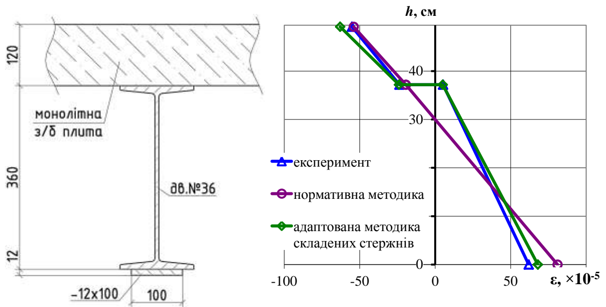
Рис. 4.35 – Порівняння відносних деформацій по висоті перерізу балок серії ПСБЗ
