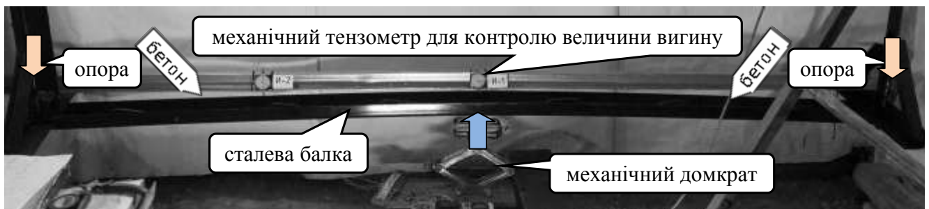
Рис. 4.21 – Попередній вигин сталеві частини перерізу балок серії ПСБ1 і ПСБ2
