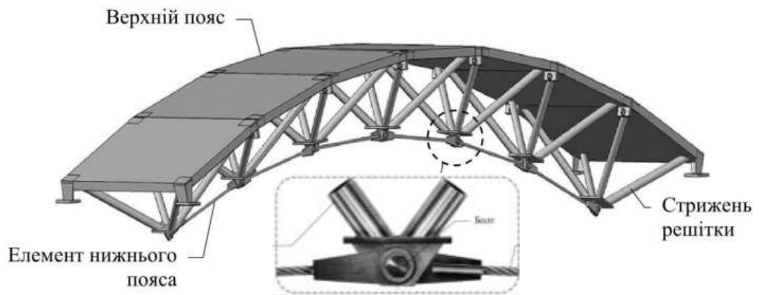
Рис. 1.19 – Загальний вигляд фрагменту просторового структурно-вантового криволінійного сталезалізобетонного покриття [197; 341]
