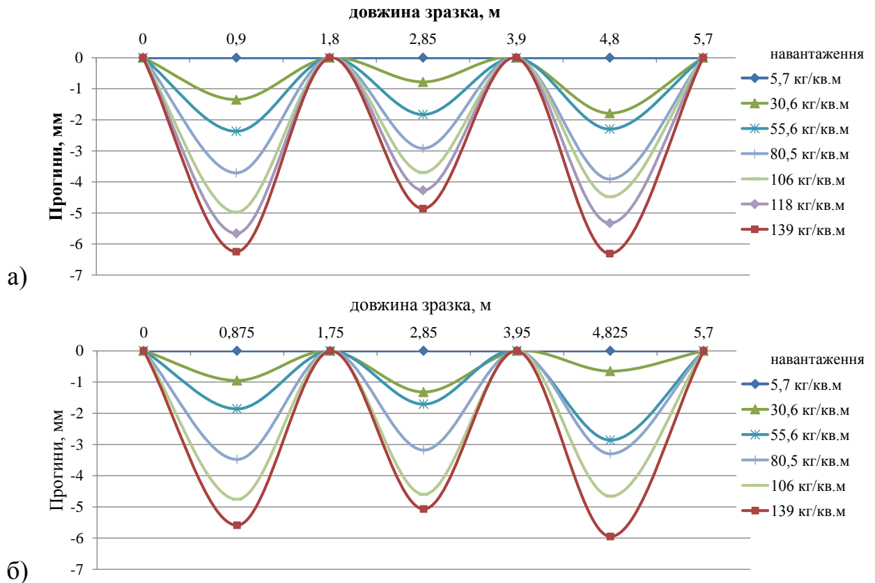
Рис. 5.20 – Зміна прогинів по довжині профільованого настилу К35-0,5:
