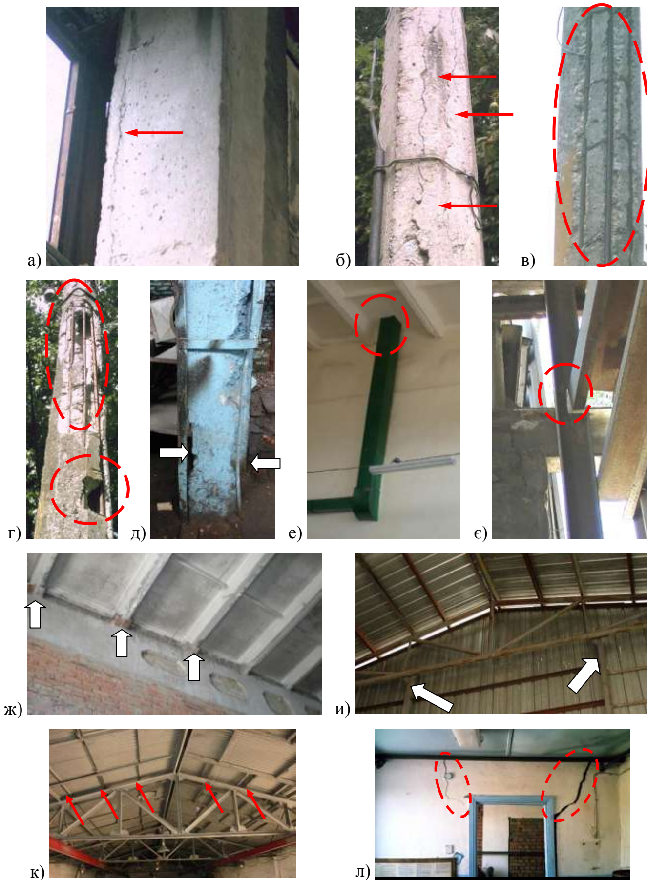
Рис. 2.15 – Характерні пошкодження будівельних конструкцій, що приводять до небажаного перерозподілу зусиль в них
