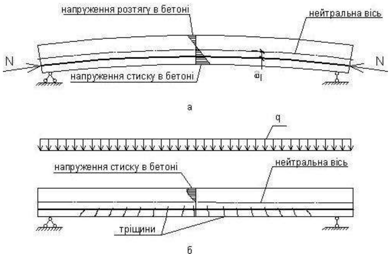
Рис. 1.33 – Принцип створення попередніх напружень у залізобетоні [144]:
