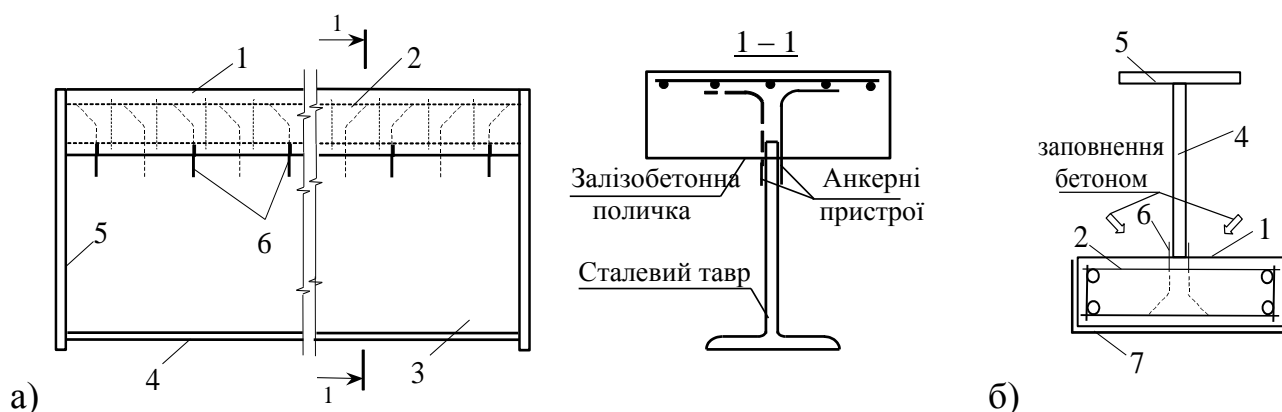
Рис. 1.15 – Сталезалізобетонна двотаврова балка із залізобетонним верхнім поясом та тавровою сталевію частиною [201]: а) будова; б) бетонування
