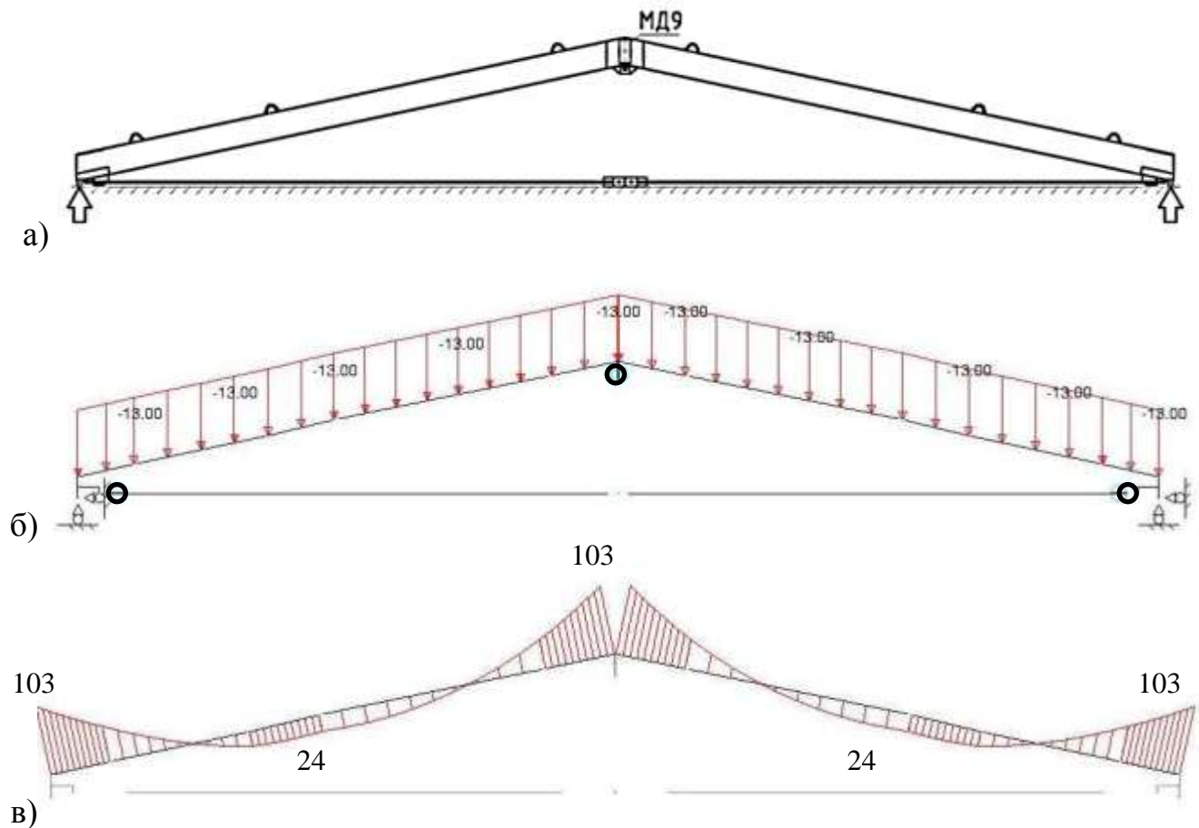
Рис. 6.18 – Демонтаж середньої опори з шарнірно нерухомими крайніми опорами та шарнірним гребневим вузлом: а) схема розташування опор; б) розрахункова схема; в) епюра згинальних моментів, кНм
