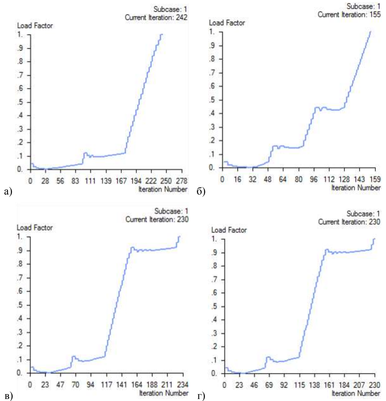
Рис. 7.20 – Графічна інтерпретація ходу використаного кроково-ітераційного методу розрахунку Ньютона-Рафсона сталевих балок при можливому нерівномірному просіданні суміжних колон для розрахункових випадків:
