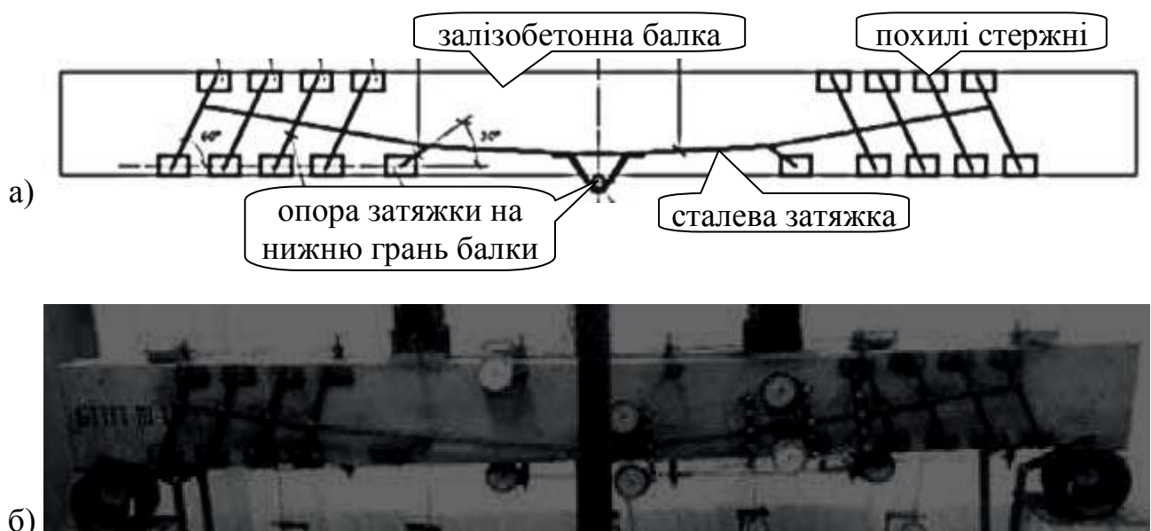
Рис. 1.2 – Конструкція регульовано-напруженої з/б балки: а) схема розташування системи поздовжньо-поперечних затяжок; б) фото під час випробування [215]
