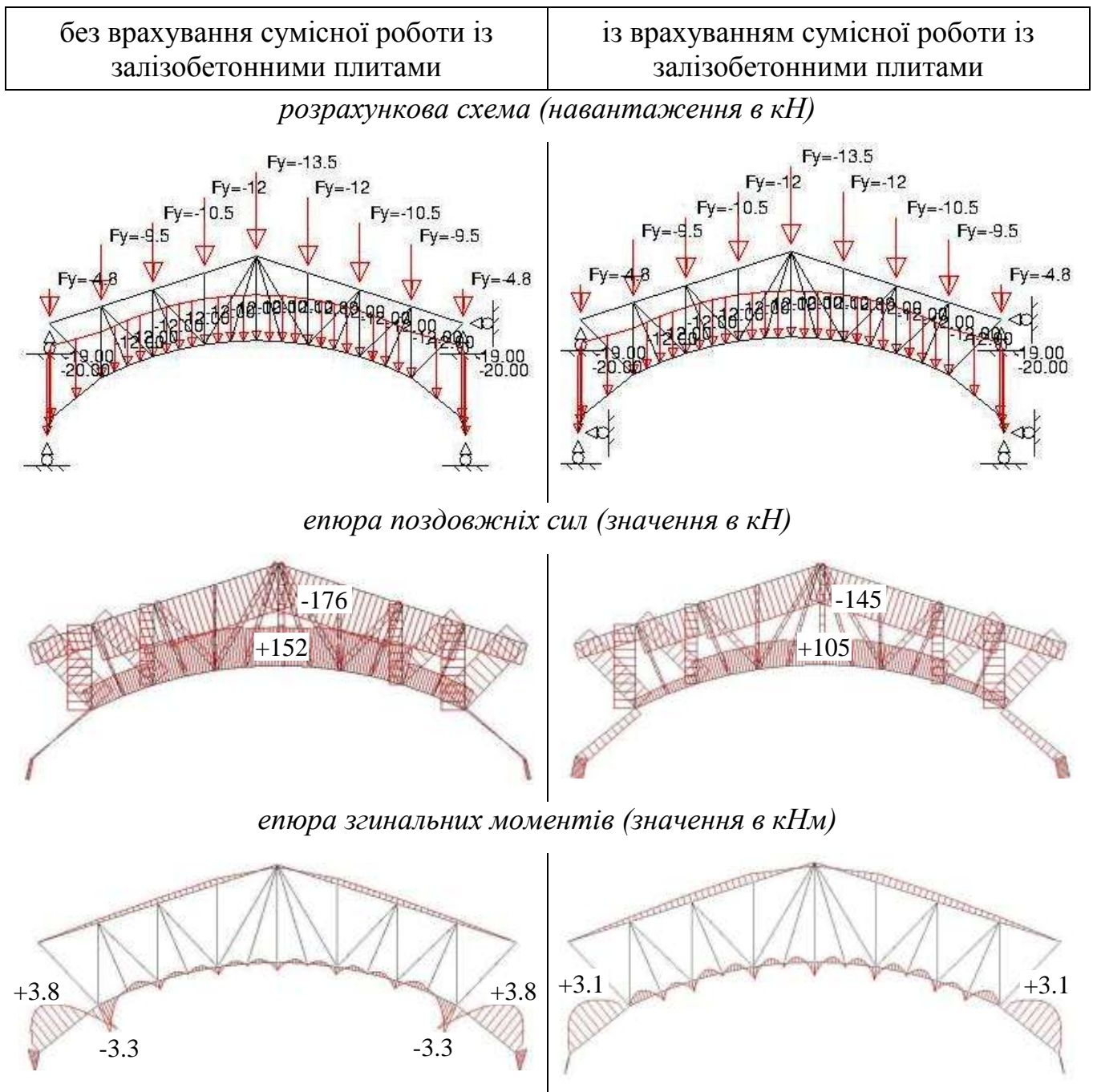
Рис. 6.24 – Розрахункова схема та епюри внутрішніх зусиль у сталевій фермі до та після перерозподілу зусиль
