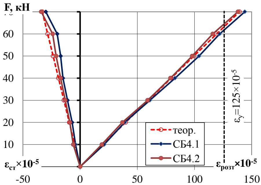
Рис. 4.14 – Приріст відносних деформацій найбільш стиснутого та розтягнутого волокон сталевій частини перерізу балок серії СБ4
