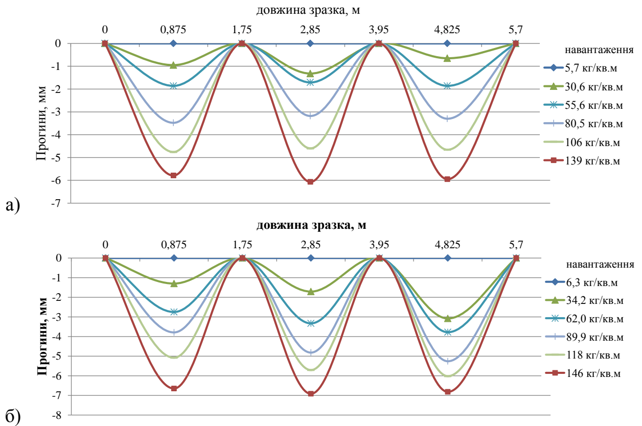
Рис. 5.21 – Зміна прогинів по довжині профільованого настилу К35-0,5:
