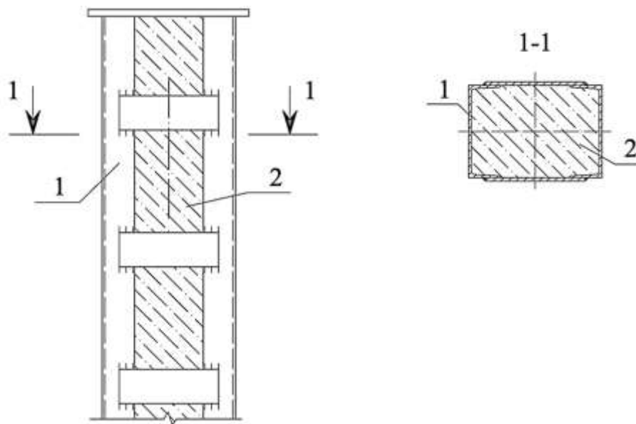
Рис. 7.21 – Підсилювана сталева колона під час бетонування
