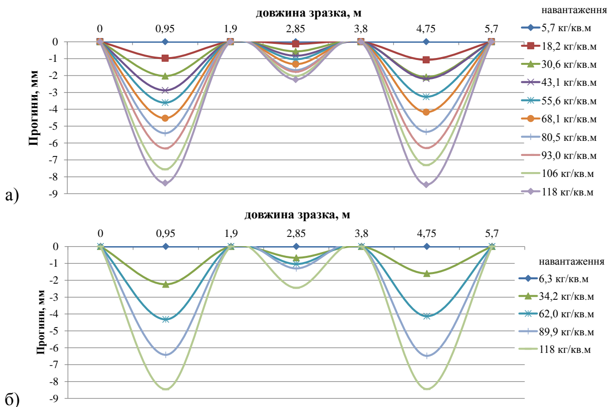
Рис. 5.19 – Зміна прогинів по довжині профільованого настилу K35-0,5:
