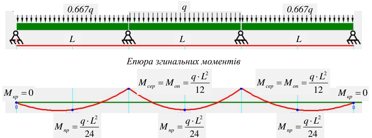
Рис. 5.5 – До визначення відношення рівномірно розподіленого навантаження шарнірної балки з трьома однаковими прольотами
