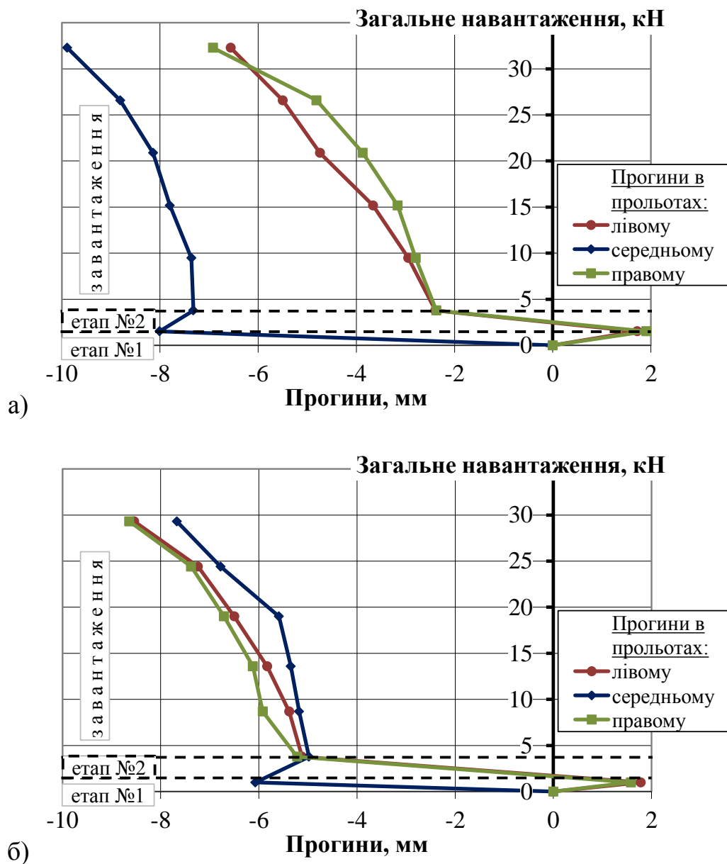
Рис. 5.34 – Розвиток прогинів у прольотах СЗБ плит на кожному етапі їх створення та в процесі завантаження: а) 1,7-2,3-1,7 СЗБП; б) 2,1-1,5-2,1 СЗБП
