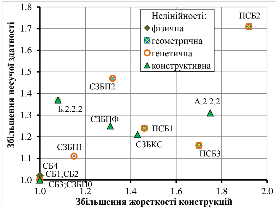
Рис. 5.27 – Відносні показники ресурсоощадності самонапружених СЗБК
