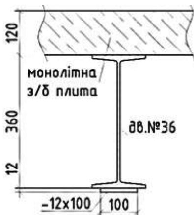
Рис. 3.19 – Поперечний переріз сталезалізобетонних балок серії ПСБЗ
