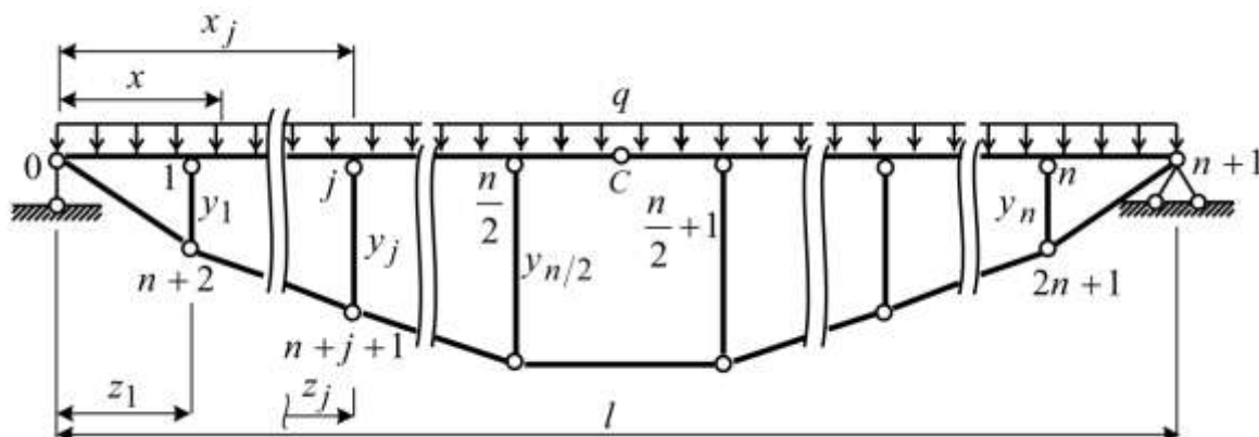
Рис. 1.21 – Схема шпренгельної балки [24]
