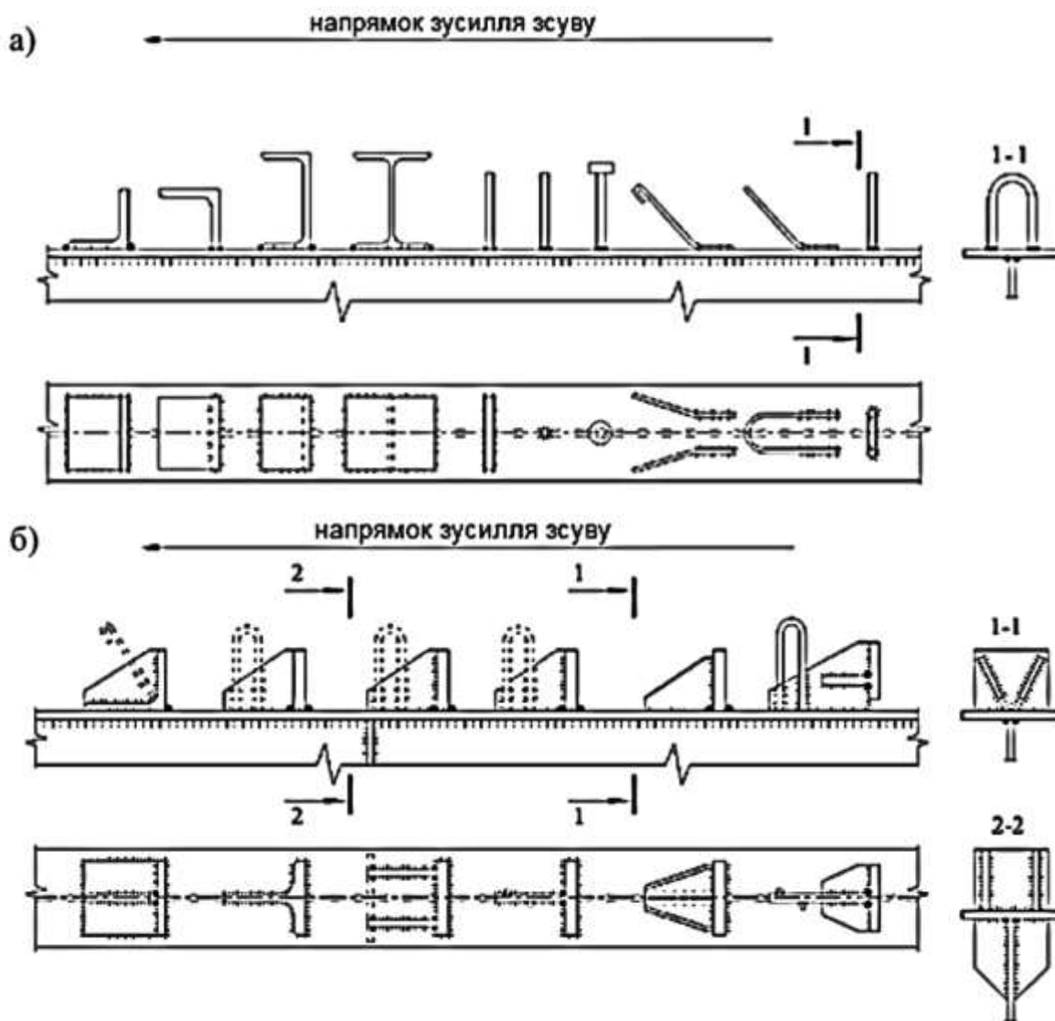
Рис. 1.41 – Найбільш розповсюджені види гнучких (а) і жорстких (б) з'єднувальних елементів компонентів сталезалізобетонного перерізу [88]
