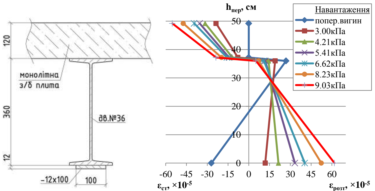
Рис. 4.34 – Зміна відносних деформацій по висоті перерізу балки серії ПСБЗ на кожному етапі навантаження
