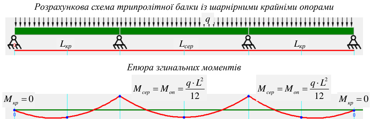
Рис. 5.2 – До визначення довжин крайніх прольотів трипролітної шарнірної балки
