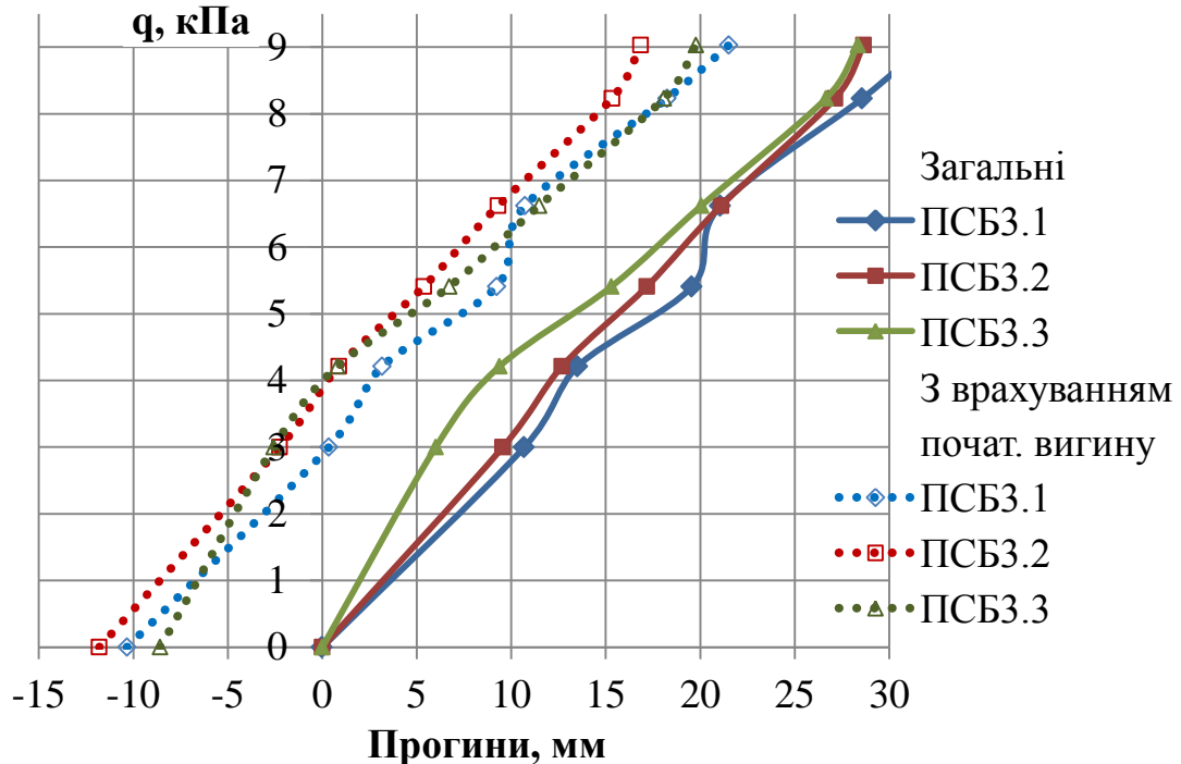
Рис. 4.37 – Зміна максимальних прогинів балок ПСБЗ
