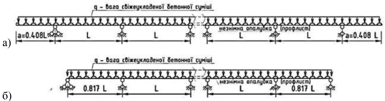
Рис. 5.4 – Оптимізовані нерозрізні багатопролітні схеми розташування опор незнімної опалубки із профліста СЗБ плит: а) консольних; б) безконсольних
