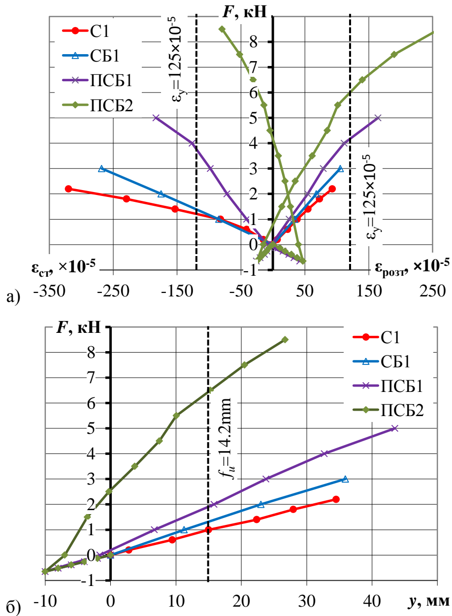
Рис. 4.26 – Порівняння розвитку відносних деформацій нормального перерізу сталеві частини (а) та прогинів (б) зразків серій СБ1, ПСБ1 і ПСБ2
