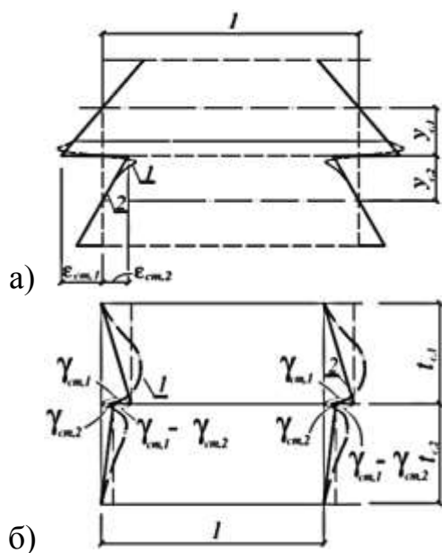
Рис. 1.46 – Розподіли відносних поздовжніх (а) та зсувних (б) деформацій по висоті двокомпонентного ЗБЕ при несумісності деформацій [300]
