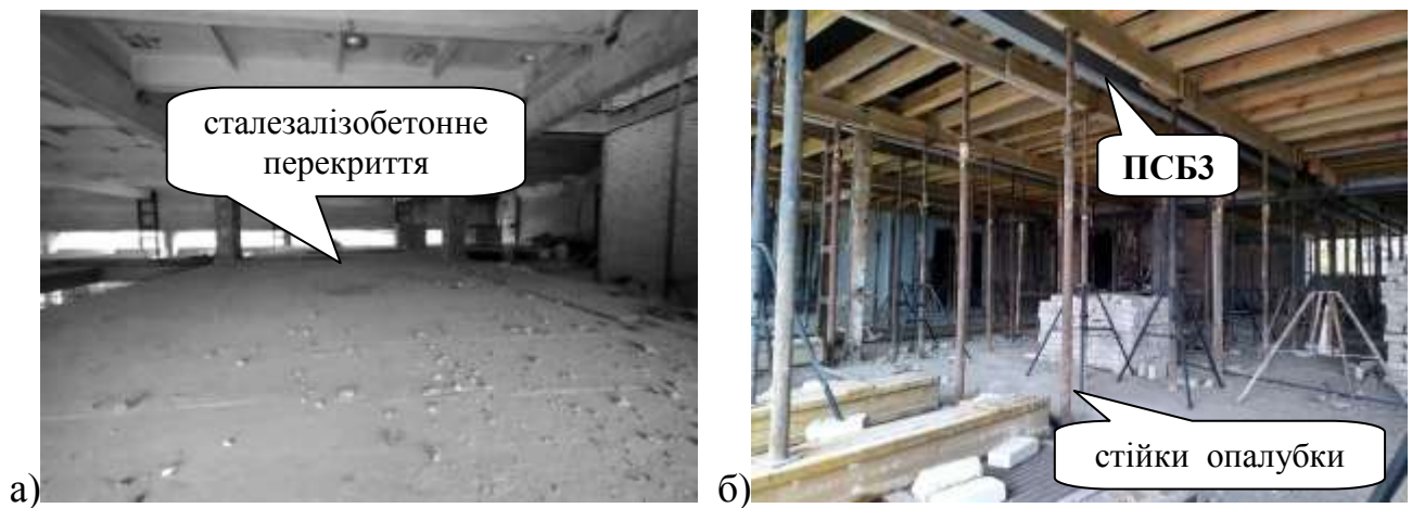
Рис. 4.29 – Загальний вигляд на сталезалізобетонне перекриття:
