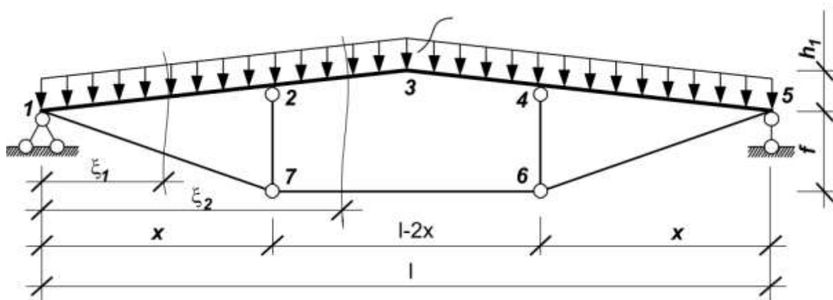
Рис. 1.20 – Розрахункова схема статично невизначної шпренгельної балки [25]
